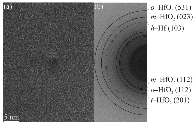
Рис. 1. (а) – ПЭМ-изображение области пленки \text{HfO}_x , подвергнутой воздействию электронного луча с \Phi = 3.0 \cdot 10^{23} \text{ см}^{-2} ( t = 15 мин), и соответствующая картина дифракции (б)
