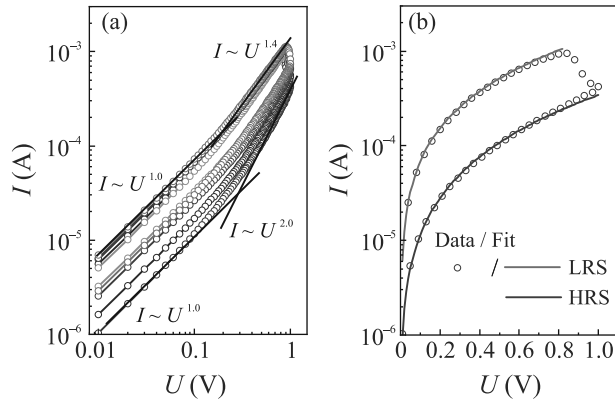
Рис. 4. (Цветной онлайн) (a) – ВАХ мемристора TaN/HfO x /Ni, полученного под воздействием электронного луча при \Phi = 2.0 \cdot 10^{23} \text{ см}^{-2} ( t = 10 мин), в двойном логарифмическом масштабе и (b) – аппроксимация его экспериментальных ВАХ (точки) для низко- и высокоомного состояний (LRS и HRS, соответственно) модельными (линии)
