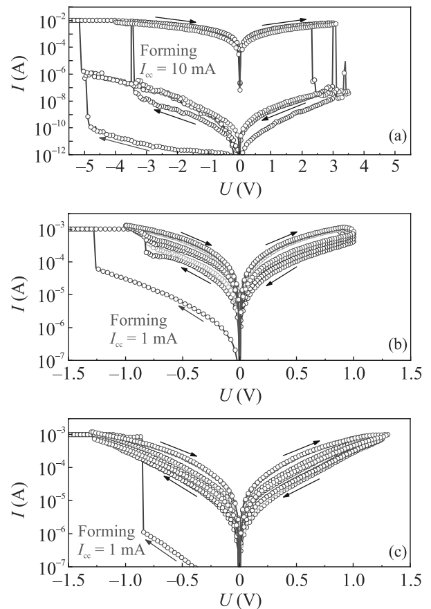
Рис. 2. (Цветной онлайн) ВАХ формовки и резистивного переключения мемристоров \text{TaN}/\text{HfO}_x/\text{Ni} , полученных при \Phi = 0 (а), 2.0 \cdot 10^{23} \text{ см}^{-2} (б) и 3.0 \cdot 10^{23} \text{ см}^{-2} (с). Стрелками показано направление развертки напряжения
