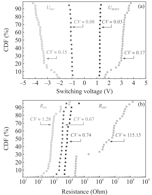
Рис. 3. (Цветной онлайн) Функции распределения напряжений переключения (а) и сопротивлений (б) мемристоров \text{TaN}/\text{HfO}_x/\text{Ni} ( x = 1.81 ), слой оксида которых подвергался воздействию электронного луча при \Phi = 2.0 \cdot 10^{23} \text{ см}^{-2} ( t = 10 мин) и без него (сплошные и пустые точки, соответственно)
