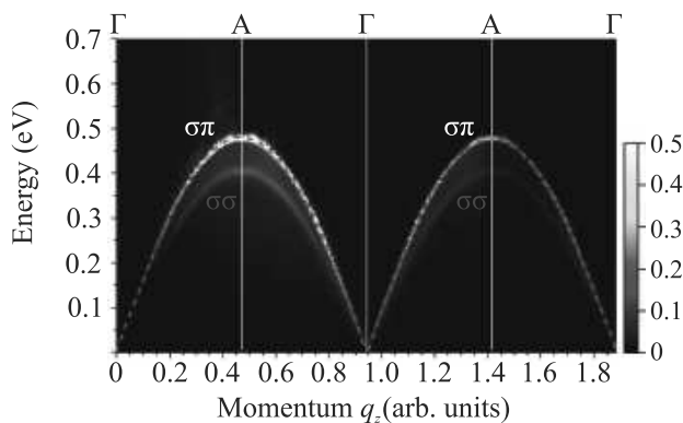
Рис. 5. (Цветной онлайн) Спектр акустического плазмона \omega_{\sigma\pi}^2 = B \sin^2(q_z d) в слоистом металле \text{MgB}_2 в направлении z , перпендикулярном базальной плоскости [33]. Спектр практически линейен в окрестностях точек q_z d \rightarrow n\pi , где n = 0, 1, \dots ; d – межплоскостное расстояние
