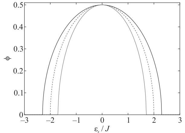
Рис. 1. (Цветной онлайн) Зависимость экситонного параметра порядка \phi от величины расщепления \varepsilon_S , полученная в приближении среднего поля при T = 0 без учета (красная штриховая линия, g_1 = 0, g_2 = 0 ), с учетом недиагонального (синяя сплошная линия, g_1 = 0, g_2 = 1.25J ) и диагонального (зеленая сплошная линия, g_1 = 1.25J, g_2 = 0 ) электрон-фононного взаимодействия. Расчеты выполнены для следующего набора параметров: z = 4, J = 28 К, J''_{ex} = -0.5J
