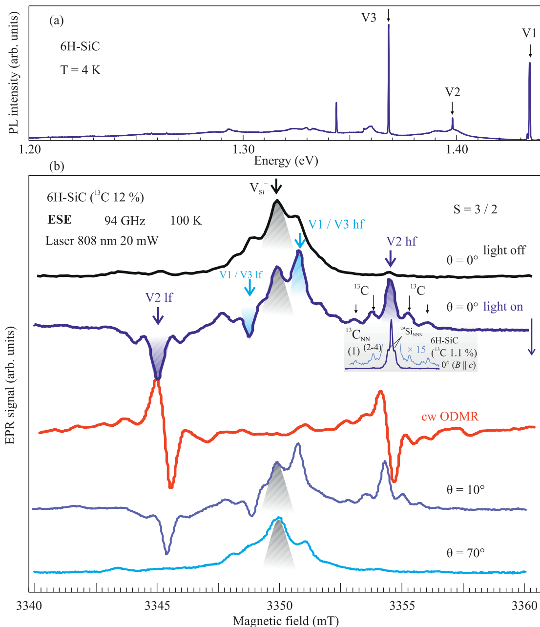
Рис. 1. (Цветной онлайн) (a) – Линии ФЛ V1, V2 и V3 центров в кристалле 6H-SiC, длина волны оптического возбуждения 795 нм. (b) – Зарегистрированные по ЭСЭ на частоте 94 ГГц спектры ЭПР кватерных спиновых центров в нескольких ориентациях кристалла 6H-SiC, обогащенного изотопом ^{13}\text{C} до 12 %, в магнитном поле при непрерывном оптическом лазерном возбуждении, за исключением верхнего спектра, который был измерен в темноте. Спектры были измерены в ориентациях \theta = 0^\circ ( B \parallel c ), \theta = 10^\circ и \theta = 70^\circ . Линии V2 и V1/V3 отмечены стрелками, видно, что при оптическом возбуждении низкополевые сигналы V2 и V1/V3 центров имеют инвертированную фазу, что обусловлено инверсной населенностью спиновых уровней, приводящей к микроволновому излучению, т.е. мазерному эффекту. Центральная линия, помеченная черным цветом на всех спектрах, не изменяется, как при оптическом возбуждении, так и при изменении ориентации кристалла. На вставке приведен спектр ЭПР V2 центров, зарегистрированный в кристалле 6H-SiC с природным содержанием изотопов. Красным цветом представлен спектр ОДМР, зарегистрированный в непрерывном режиме (cw) в том же образце, что и спектры ЭСЭ в ориентации, близкой к B \parallel c
