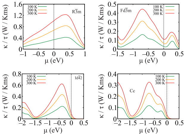
Рис. 6. (Цветной онлайн) Зависимость электронной теплопроводности, деленной на время релаксации, от химического потенциала при температурах 100, 200 и 300 К для R\bar{3}m , \text{Fd}\bar{3}m , I\bar{4}2d и Cc структур
