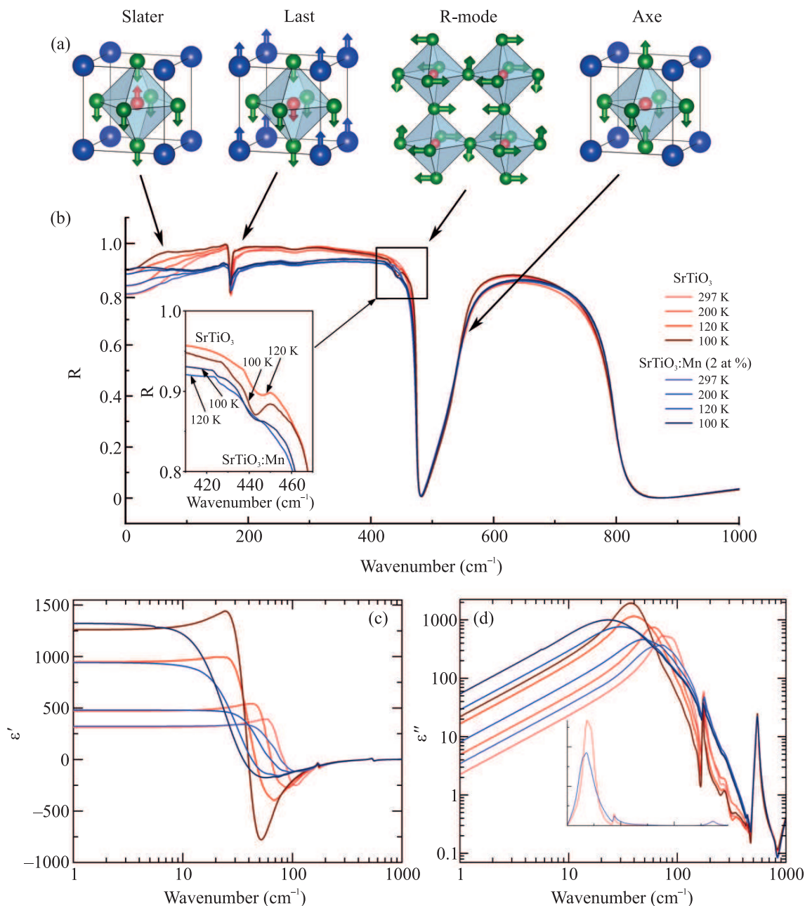
Рис. 1. (Цветной онлайн) (a) – Нормальные координаты, соответствующие симметрично-разрешенным в ИК спектрах кристаллов SrTiO 3 модам (ТО компонентам мод с симметрией F_{1u} ). Появление R-моды возможно только при температурах ниже антиферодисторсионного перехода. Атомы Sr – синие (для R-моды не показаны), Ti – красные, O – зеленые. (b) – ТГц-ИК спектры коэффициента отражения кристаллов SrTiO 3 и SrTiO 3 :Mn (2 ат. %), измеренные при нескольких температурах. Рамками показаны спектральные особенности, соответствующие различным типам колебаний, как указано стрелками. Вставка: спектры коэффициента отражения в интервале 410–470 см -1 . Появление аномалии при 442 см -1 соответствует ИК-активной компоненте R-моды, возникающей при антиферодисторсионном переходе. (c), (d) – Спектры действительной (c) и мнимой (d) частей диэлектрической проницаемости кристаллов SrTiO 3 и SrTiO 3 :Mn (2 ат. %), полученные методом Крамерс–Крониг анализа широкодиапазонных спектров отражения R(\nu) , как описано в тексте. Вставка на панели (d): спектры \epsilon''(\nu) при температуре 297 K в линейном масштабе по обоим осям
