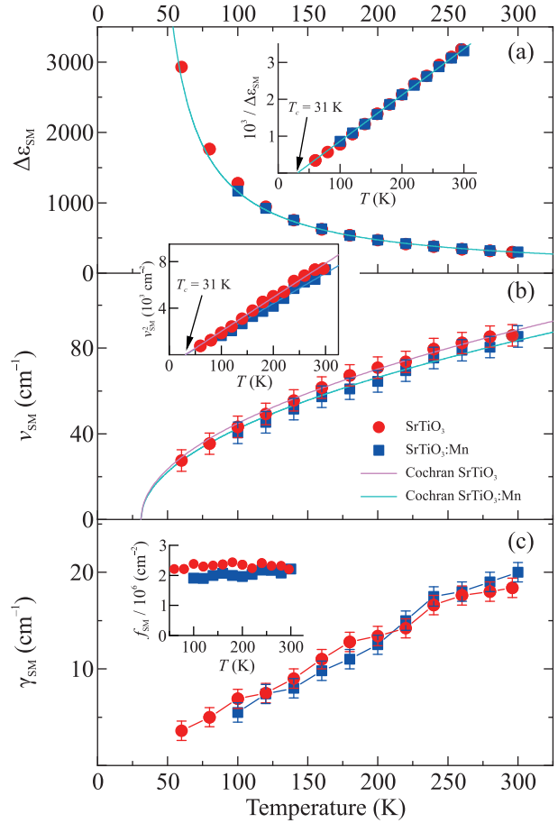
Рис. 3. (Цветной онлайн) Температурные зависимости параметров сегнетоэлектрической мягкой моды в монокристаллах \text{SrTiO}_3 и \text{SrTi}_{1-x}\text{Mn}_x\text{O}_3 ( x = 2\text{ ат.}\% ): диэлектрического вклада (a), обратной величины диэлектрического вклада (панель (a), вставка), частоты (b), квадрата частоты (панель (b), вставка), затухания (c), силы осциллятора (панель (c), вставка). Линии на панели (a) и на вставке на панели (a) соответствуют выражению Кюри-Вейсса ((5) в тексте) с температурой Кюри-Вейсса T_C = 31\text{ К} . Линии на панели (b) и на вставке на панели (b) соответствуют выражению Кохрана ((1) в тексте) с температурой Кюри-Вейсса T_C = 31\text{ К}
