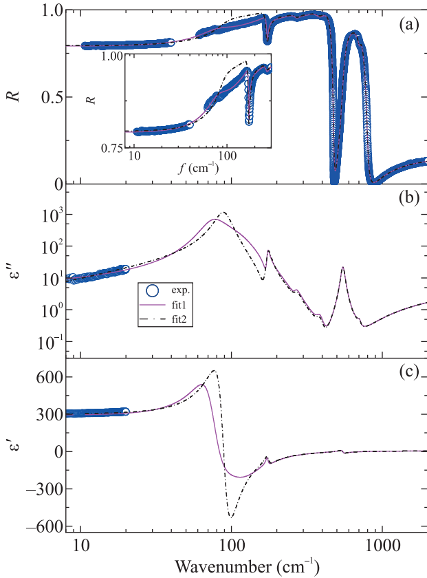
Рис. 2. (Цветной онлайн) ТГц-ИК спектры коэффициента отражения (a), мнимой (b) и действительной (c) частей диэлектрической проницаемости кристалла \text{SrTiO}_3\text{:Mn} при 297 К. ТГц данные на частотах ниже 20\text{ см}^{-1} (точки на панелях (b), (c)) получены путем прямых измерений на ТГц спектрометре с временным разрешением. Линии соответствуют одновременной обработке методом наименьших квадратов ТГц спектров \varepsilon'(\nu) и \varepsilon''(\nu) и ИК спектров коэффициента отражения R(\nu) , как описано в тексте: розовая, fit1 на рисунке, (штрихпунктирная, fit2 на рисунке) линия отвечает обработке спектров с использованием четырехпараметрической фактаризованной модели с учетом (без учета) низкочастотного возбуждения, расположенного ниже мягкой сегнетоэлектрической моды; соответствующие результаты показаны в деталях на вставке на панели (a)
