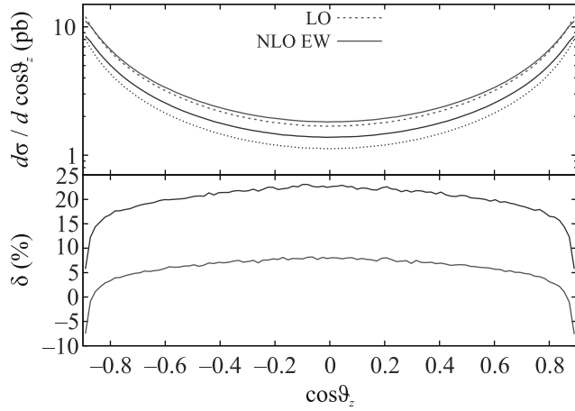
Рис. 4. (Цветной онлайн) Сечения в борновском и однопетлевом (по частям) приближениях, а также относительные поправки при энергии \sqrt{s} = 250 ГэВ с поляризованными начальными пучками
