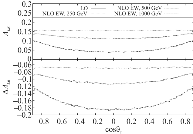
Рис. 8. (Цветной онлайн) Распределение лево-правой асимметрии A_{LR} по \cos\vartheta_Z в борновском и однопетлевом приближении при энергиях \sqrt{s} = 250, 500, 1000 ГэВ в схеме \alpha(0)
