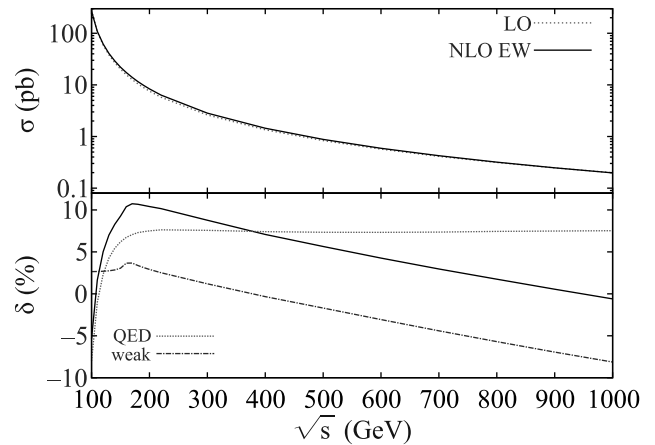
Рис. 7. (Цветной онлайн) Сечения в борновском и однопетлевом приближениях для неполяризованных начальных пучков и относительные поправки (по частям) как функция энергии в системе центра масс
