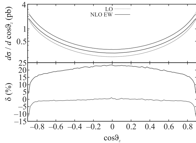
Рис. 5. (Цветной онлайн) То же самое, что и на рис. 4, но для энергии \sqrt{s} = 500 ГэВ
