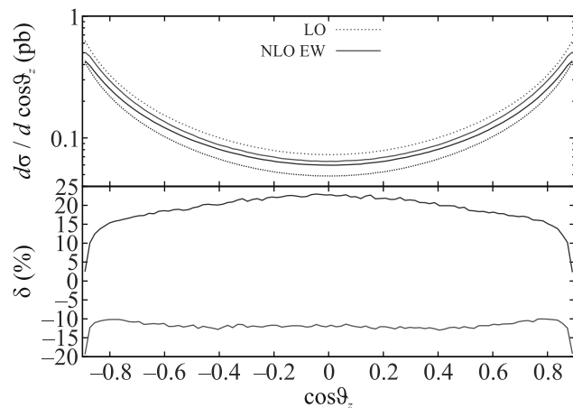
Рис. 6. (Цветной онлайн) То же самое, что и на рис. 4, но для энергии \sqrt{s} = 1000 ГэВ
