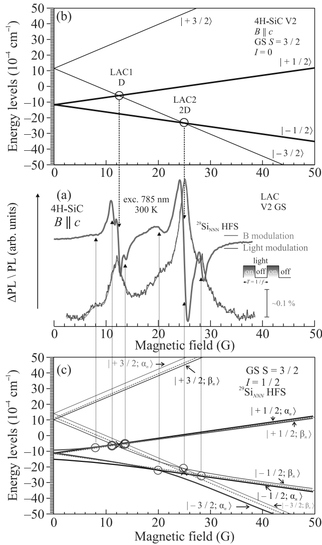
Рис. 2. (Цветной онлайн) (а) – Сигналы LAC, зарегистрированные по изменению интенсивности ФЛ спиновых центров V2. Верхний спектр (синий цвет) показывает сигналы LAC, зарегистрированные с низкочастотной модуляцией магнитного поля; нижний спектр (красный цвет) показывает сигналы LAC, зарегистрированные с использованием низкочастотной модуляции интенсивности возбуждающего света лазера. (б) – Схема энергетических уровней в магнитном поле для четных изотопов кремния. Уровни, соответствующие состояниям M_S = \pm 1/2 , отмечены более толстыми линиями, чтобы подчеркнуть преимущественное заселение этих уровней в результате оптического выстраивания. Кружками обозначены точки LAC в основном состоянии. (с) – Схема энергетических уровней в магнитном поле с учетом сверхтонких взаимодействий с одним ядром изотопа ^{29}\text{Si} . Пунктиром для сравнения приведены энергетические уровни для I = 0 , крестиками указаны две соответствующие точки LAC
