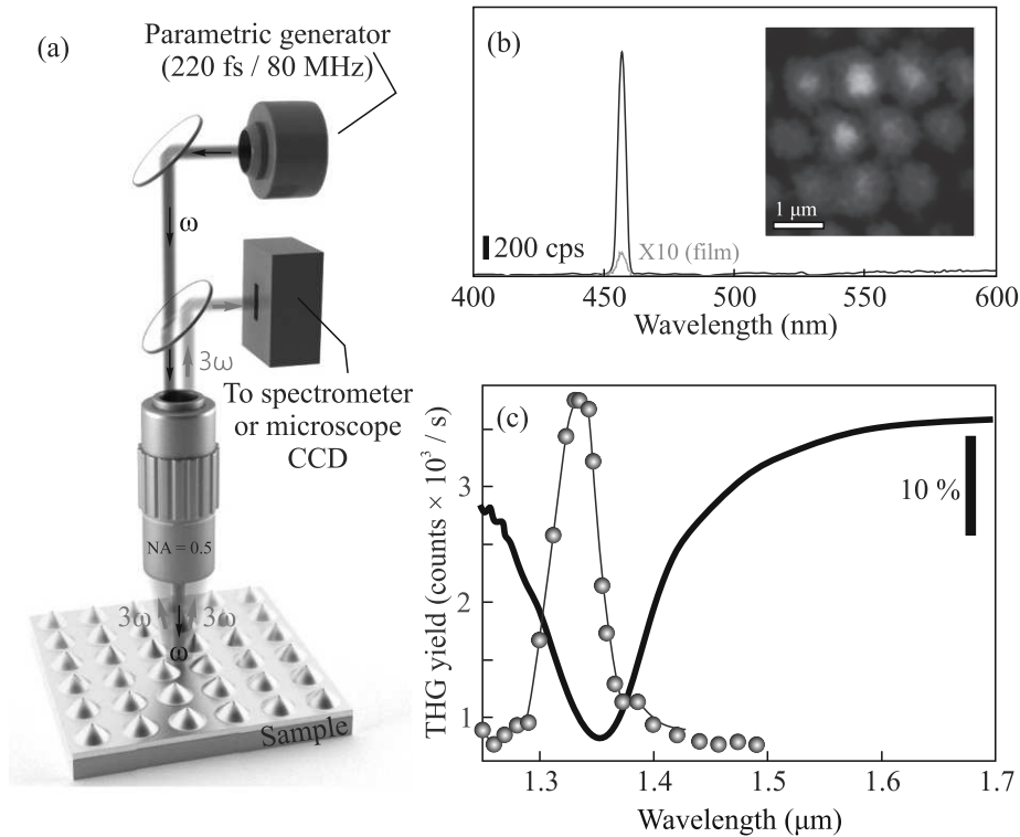
Рис. 3. (Цветной онлайн) (а) – Схема накачки и регистрации сигнала ГТГ от плазмонных метаповерхностей, состоящих из массивов полых нановыпуклостей на поверхности золотой пленки ( d = 0.9 \mu\text{м} ; E = 0.95 \text{ нДж} ). (б) – Типичный спектр ГТГ указанных наноструктур в сравнении с аналогичным спектром, измеренным от ровной поверхности золотой пленки. Длина волны и средняя мощность излучения накачки наноструктур на основной гармонике – 1370 \text{ нм} и 40 \text{ мВт} , соответственно. На вставке приведено микроскопическое изображение плазмонной метаповерхности в режиме ГТГ. (с) – Зависимость интенсивности сигнала ГТГ от длины волны накачки на основной гармонике (синие маркеры), а также спектр Фурье-ИК отражения соответствующей метаповерхности (серая кривая)
