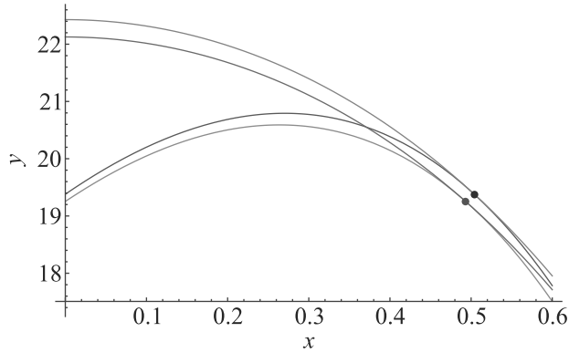
Рис. 1. (Цветной онлайн) Функция y = m_s/m_d от x = m_u/m_d в NLO приближении для случая, когда выполняется низкоэнергетическая теорема Гассера-Лойтвилера (эллипс, верхние кривые), и когда выполняются массовые формулы (кубика, нижние кривые). Поскольку теорема Дашена нарушена, для каждого из случаев изображены две кривые, охватывающие интервал \epsilon = 0.79(6) . Кривые имеют общую касательную в точке (r_x, r_y) . Воображаемая горизонтальная линия y = r_y пересекает кубическую кривую в точках (r_x, r_y) и (0, r_y)
