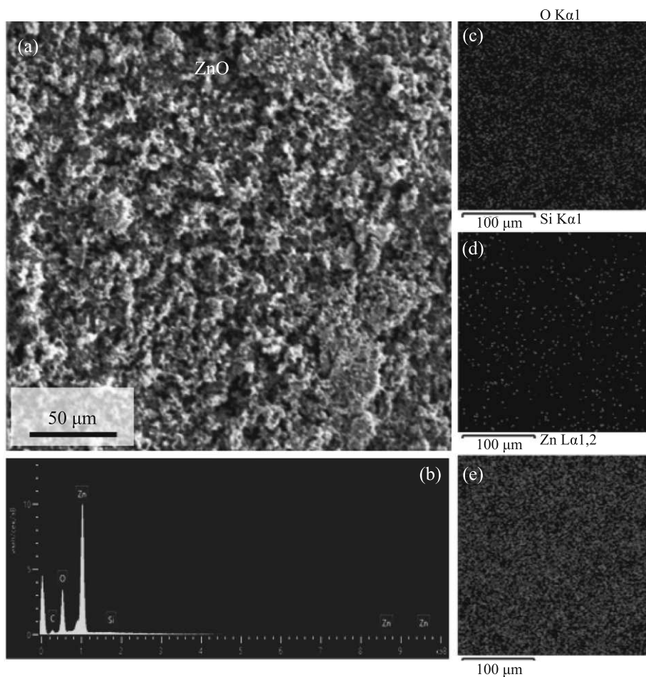
Рис. 4. (Цветной онлайн) (a) — СЭМ-изображение поверхности пленки ZnO; (b) — соответствующий энергодисперсионный спектр; (c)–(e) — карты распределения элементов в выбранной области.
