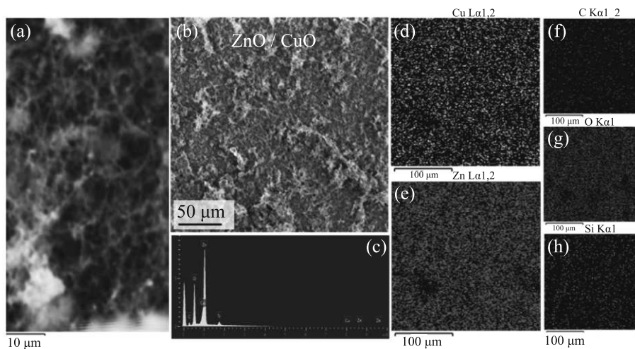
Рис. 5. (Цветной онлайн) (a), (b) — СЭМ-изображение поверхности пленки ZnO/CuO при различных увеличениях; (c) — соответствующий энергодисперсионный спектр; (d)–(h) — карты распределения элементов в выбранной области.
