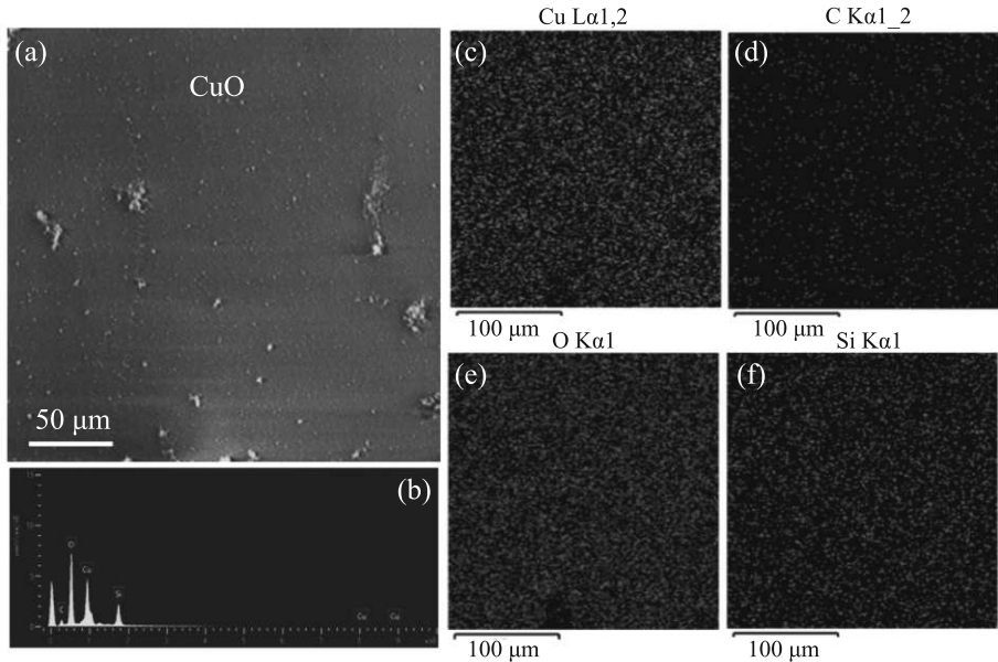
Рис. 3. (Цветной онлайн) (а) – СЭМ-изображение поверхности пленки CuO; (б) – соответствующий энергодисперсионный спектр; (с)–(f) – карты распределения элементов в выбранной области
