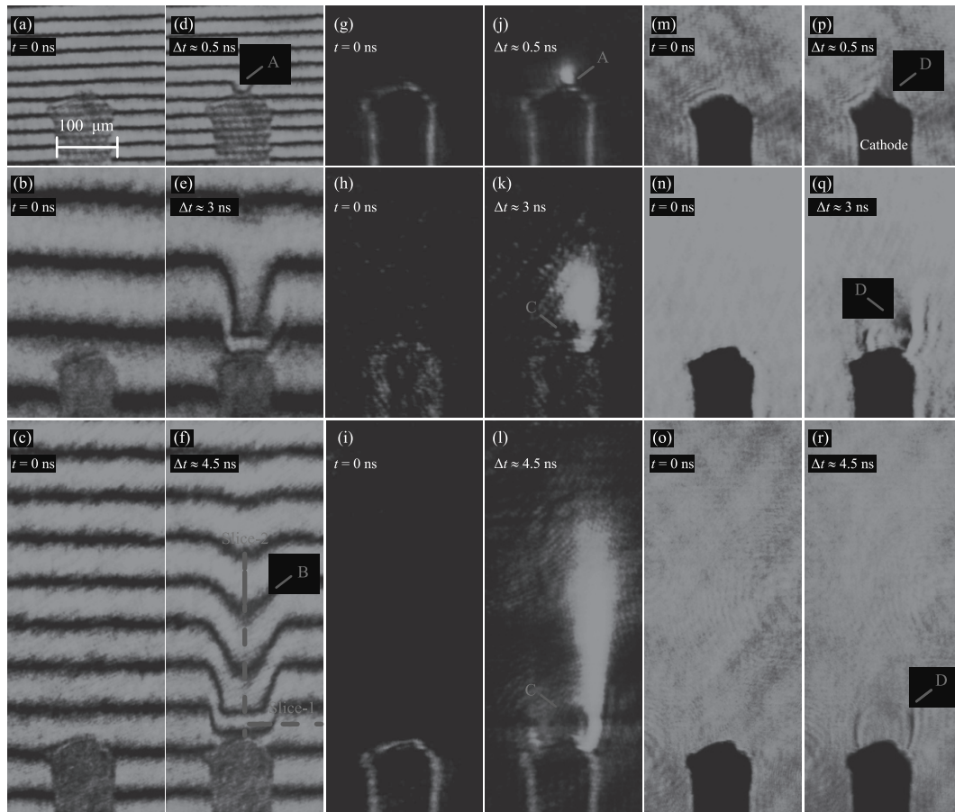
Рис. 3. (Цветной онлайн) Интерферограммы (a)–(f), шlierен-изображения (g)–(l) и тенеграммы (m)–(r), зарегистрированные в одиночном выстреле до ( t = 0 нс) разряда и в различные моменты времени ( \Delta t = t - t_{br} ) после пробоя промежутка ( t_{br} \approx 5 нс). Буквами на рисунках обозначены: А – катодное пятно, В – развивающийся искровой канал, С – сферическая область плазмы с высоким градиентом электронной плотности, D – зоны резкого падения контраста изображения
