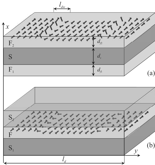
Рис. 1. (Цветной онлайн) Схематическое изображение F/S/F (a) и S/F/S (b) систем, в которых один из ферромагнитных слоев разделен полосовые домены стенками Блоха (a) или Нееля (b)
