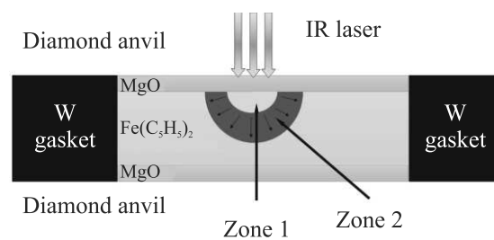
Рис. 6. (Цветной онлайн) Схема лазерного нагрева ферроцена \text{Fe}(\text{C}_5\text{H}_5)_2 в КВД. Диаметр сфокусированного лазерного пятна составлял 25–30 мкм
