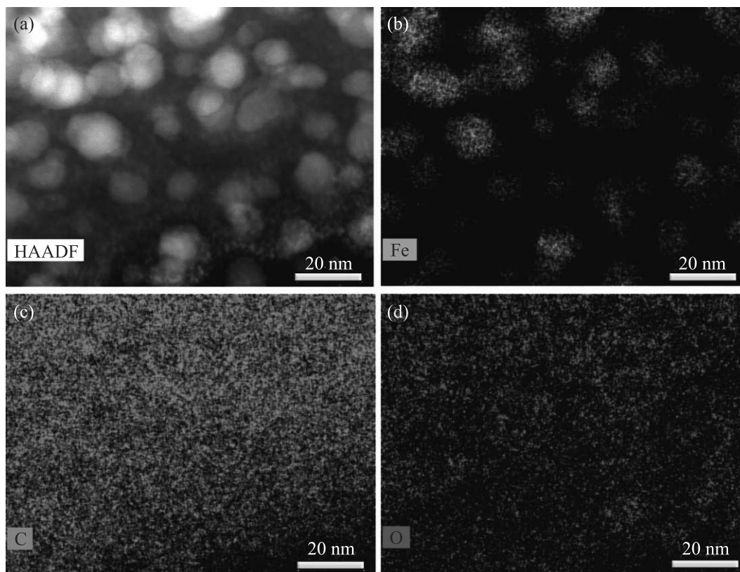
Рис. 3. (Цветной онлайн) (а) – Темнопольное ПРЭМ изображение наночастиц образца, полученное регистрацией электронов, рассеянных на большие углы. Карты распределения элементов микрообразца из КВД после ВДВТ обработки ферроцена: (b) – Fe; (c) – C и (d) – O
