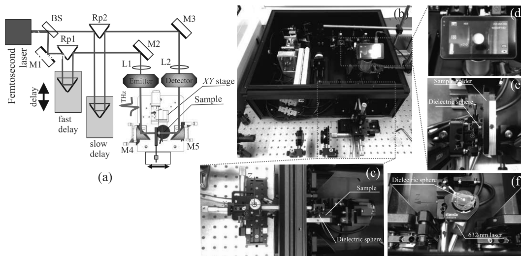
Рис. 1. (Цветной онлайн) (а), (b) – Оптическая схема и вид сверху экспериментальной установки время-разрешенного ТГц спектрометра Т-Спек (ЕКСРЛА, Вильнюс, Литва). Отдельно вынесены изображение трехкоординатного линейного транслятора (с), который служит для точного позиционирования диэлектрической сферы относительно ТГц пучка и поверхности образца, и увеличенное изображение экрана камеры (d), используемой для визуального контроля положения сферы относительно образца. (e) и (f) – Ирисовая диафрагма с диэлектрической сферой по центру
