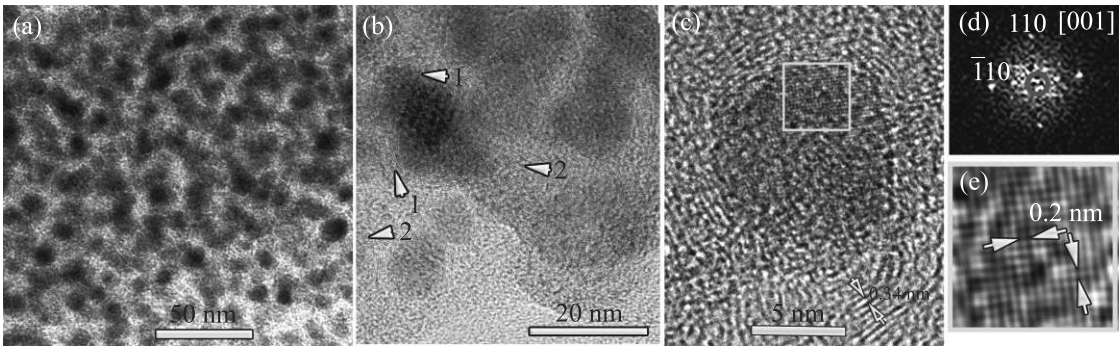
Рис. 4. (Цветной онлайн) Изображение наночастиц Fe, полученных при ВДВТ обработке ферроцена: (a) – светлпольное ПЭМ изображение; (b) – ВР ПЭМ изображение наночастиц. Стрелками с цифрами обозначены углеродные волокна, ассоциированные с наночастицами Fe (1) и располагающимися отдельно от наночастиц (2); (c) – ВРПЭМ изображение отдельной наночастицы. Квадратом выделена область анализа кристаллической решетки наночастицы. (d) – Двумерный спектр Фурье от выделенной на рис. 4с области. Спектр совпадает с электронограммой от ОЦК-Fe в проекции [001]; (e) – ВР ПЭМ изображение участка кристаллической решетки наночастицы после фильтрации
