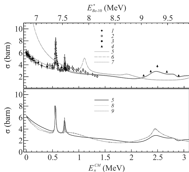
Рис. 1. Результаты расчета сечения упругого рассеяния ^9\text{Be}(n, n)^9\text{Be} . Цифрами 1–4 на рисунке обозначены результаты измерений: 1 – Lane et al. (1964); 2 – Chien et al. (1966); 3 – Lyapin et al. (1989); 4 – Levin, Cranberg (1959); цифрами 5–7 – результаты расчетов: 5 – результаты расчета с экспериментальными значениями энергий резонансов, 6 – результаты расчета с теоретически рассчитанными значениями энергий резонансов, 7 – результаты расчета с экспериментальными значениями как энергий резонансов, так и АНК; цифрами 8, 9 – оцененные сечения: 8 – оцененное сечение из базы данных ENDF/B-VII.1 [27], 9 – оцененное сечение из базы данных RUSFOND-2010 [28]
