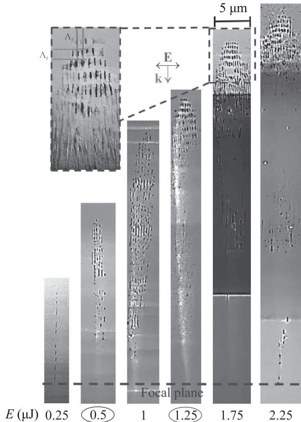
Рис. 4. (Цветной онлайн) СЭМ-визуализация эволюции поперечных сечений микротреков, записанных объективом с апертурой NA=0.45 и длительностью 0.3 пс при различных энергиях в импульсе
