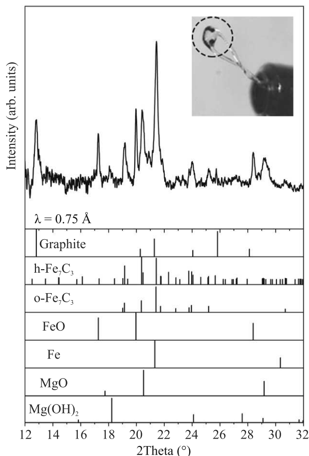
Рис. 2. (Цветной онлайн) Рентгенограмма образца и штрих диаграммы наиболее вероятных соединений. На вставке пунктиром показан микрообразец размером около 40 мкм на держателе. Штрих диаграммы построены по данным базы ICDD: графит (PDF # 00-023-0064), \alpha - \text{Fe}_7\text{C}_3 (PDF # 01-075-1499), h - \text{Fe}_7\text{C}_3 (PDF # 00-017-0333), FeO (PDF # 00-006-0615), \alpha -Fe (PDF # 00-006-0696), MgO (PDF # 00-004-0829), \text{Mg}(\text{OH})_2 (PDF # 00-044-1482).
