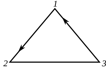
Рис. 1. Частично-ориентированный граф, соответствующий матрице A_1
