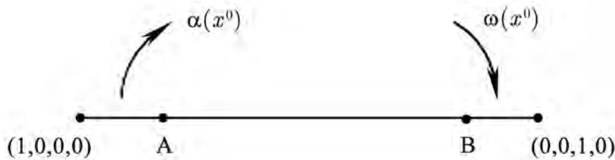
Рис. 4. Расположение множеств \alpha(x^0) и \omega(x^0)
