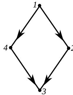
Рис. 3. Частично-ориентированный граф, соответствующий матрице A_2
