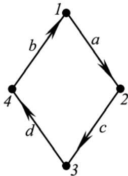
Рис. 6. Частично-ориентированный граф, соответствующий матрице A_4
