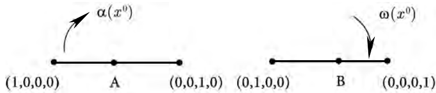
Рис. 5. Расположение множеств \alpha(x^0) и \omega(x^0) для V_3 Fig. 5. The arrangement of the sets \alpha(x^0) and \omega(x^0) for V_3
