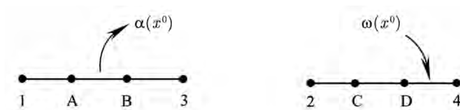
Рис. 7. Расположение множеств \alpha(x^0) и \omega(x^0) для V_4
