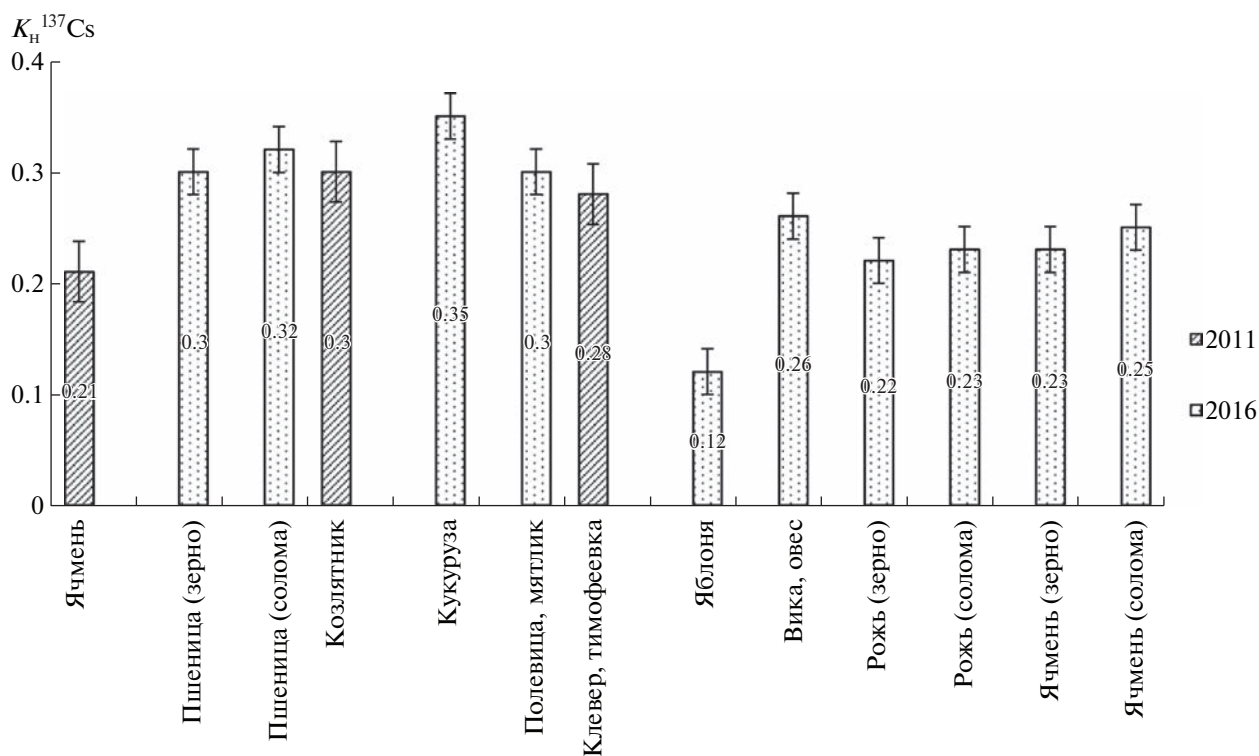
Рис. 2. Коэффициенты накопления ^{137}\text{Cs} растениями.
