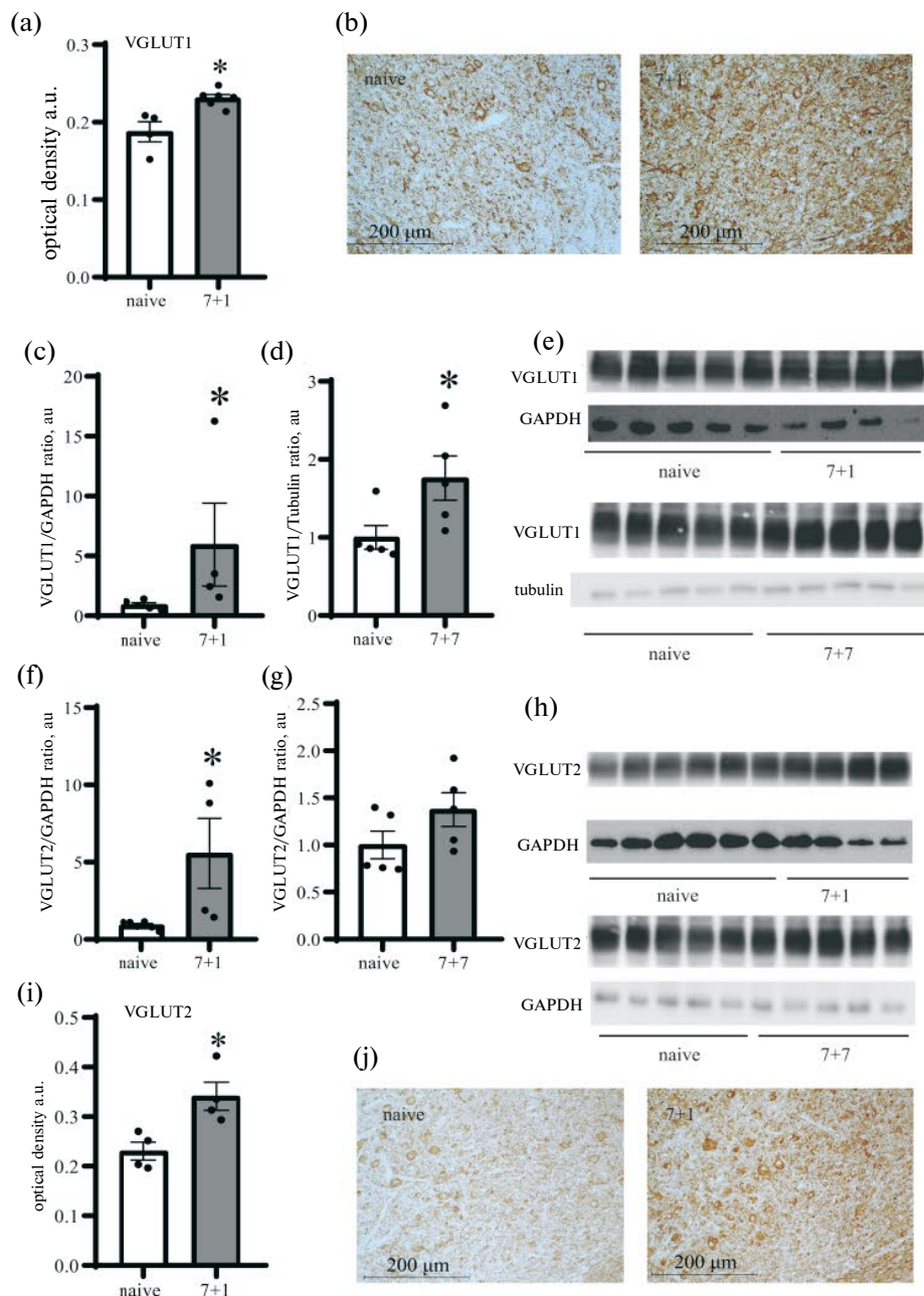
Рис. 3. Анализ содержания транспортеров глутамата VGLUT1 и VGLUT2 в НБЧ крыс линии КМ после 7-дневного киндинга: содержание белков VGLUT2 и VGLUT1 оценивали по оптической плотности VGLUT1 (a); VGLUT2 (i) иммунореактивного вещества на гистологических препаратах НБЧ. Репрезентативные изображения НБЧ: VGLUT1 (b); VGLUT2 (j). Также оценку содержания везикулярных транспортеров проводили методом Вестерн-блот анализа: VGLUT1 (c, d); VGLUT2 (f, g). Графики показывают оптическую плотность иммунопозитивного вещества, произвольные единицы (а. у.). Репрезентативные изображения иммуноблотов (e) и (h) соответственно. Данные представлены как среднее \pm SEM. * – p < 0.05 по сравнению с контролем.
