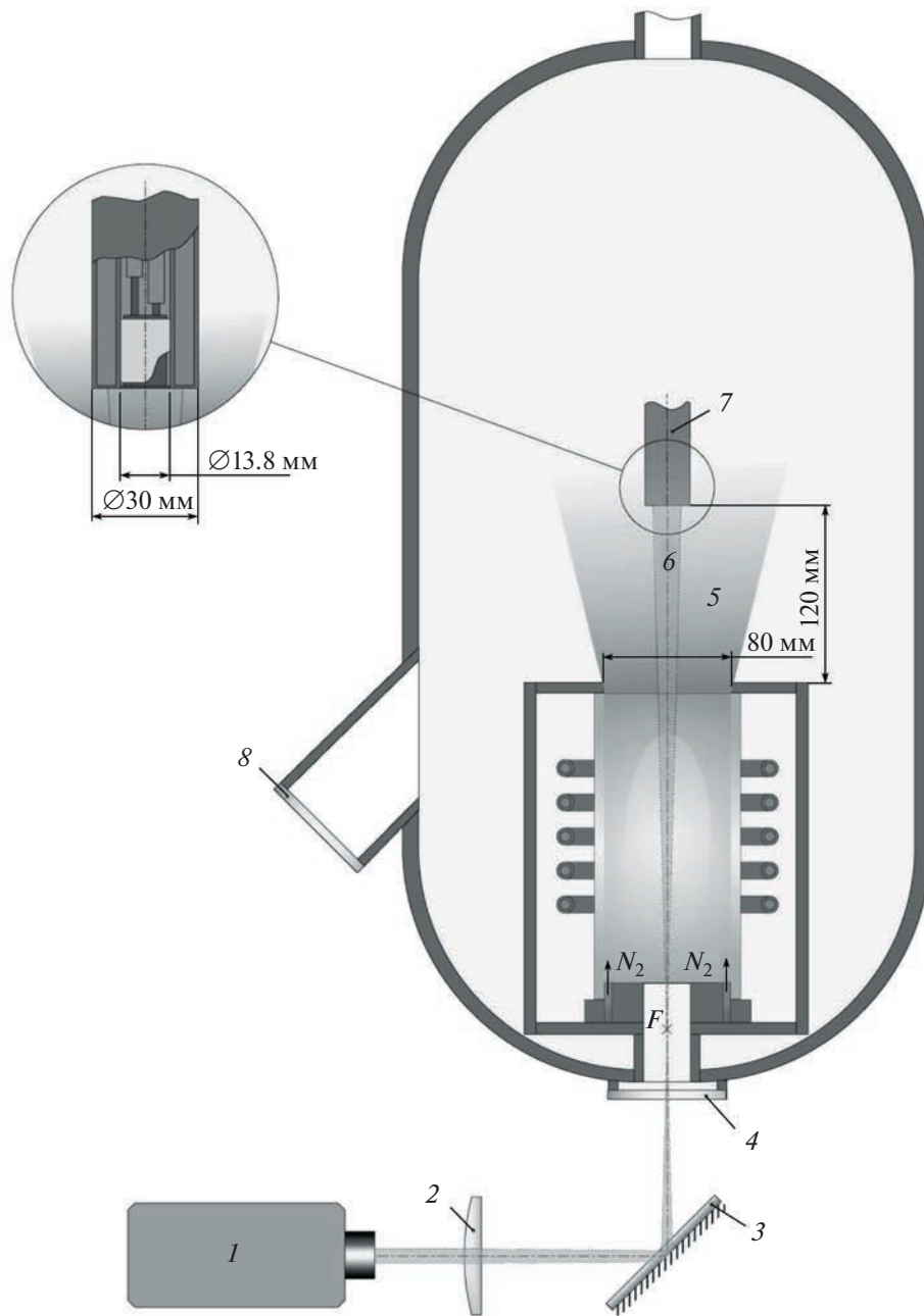
Рис. 1. Схема ВЧ-плазматрона ВГУ-4, дополнительно оснащенного источником лазерного излучения: 1 – импульсный волоконный лазер; 2 – линза; 3 – поворотное зеркало; 4 – кварцевое окно; 5 – дозвуковая струя плазмы азота; 6 – лазерный луч; 7 – медная водоохлаждаемая модель с калориметрическим датчиком; 8 – смотровое окно.
