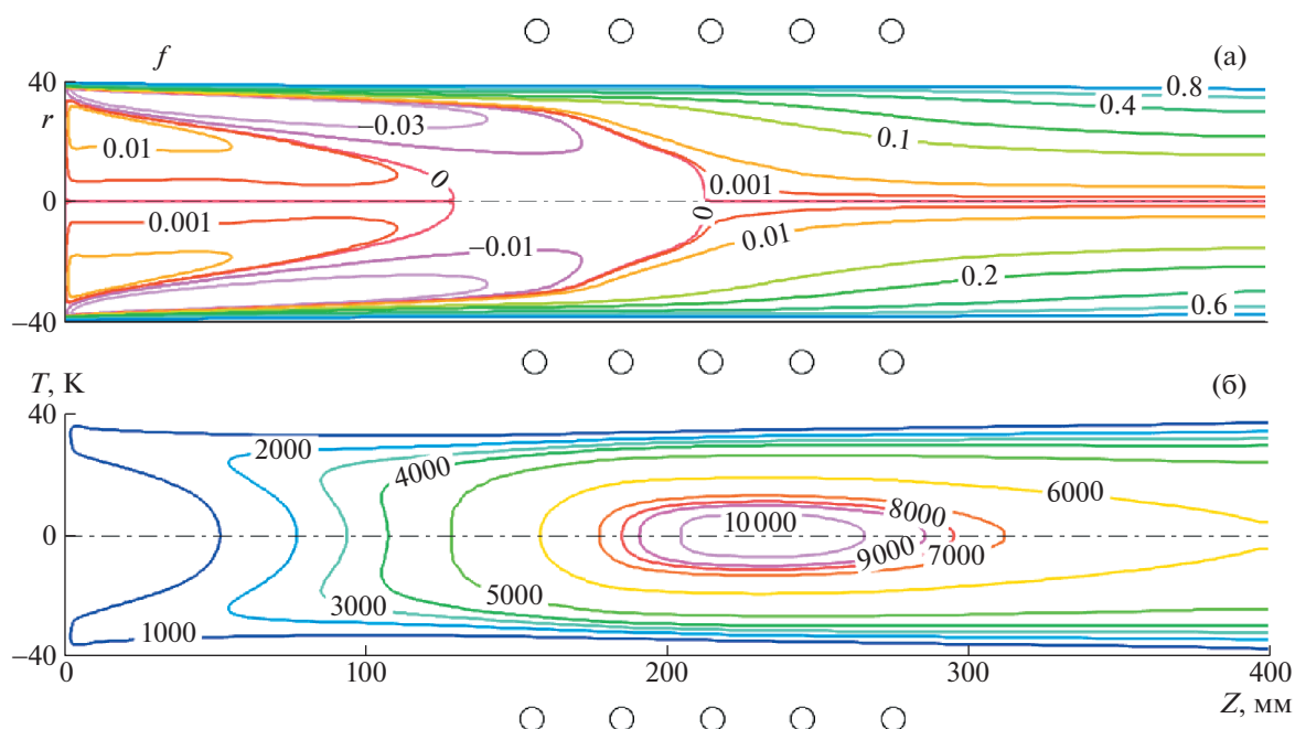
Рис. 4. Изолинии безразмерной функции тока (а) и изотермы (б) плазмы азота в разрядном канале установки ВГУ-4 для p = 1 \times 10^4 Па, N_{a.p.} = 22 кВт, N_{pl} = 12.65 кВт, G = 2.4 г/с.
