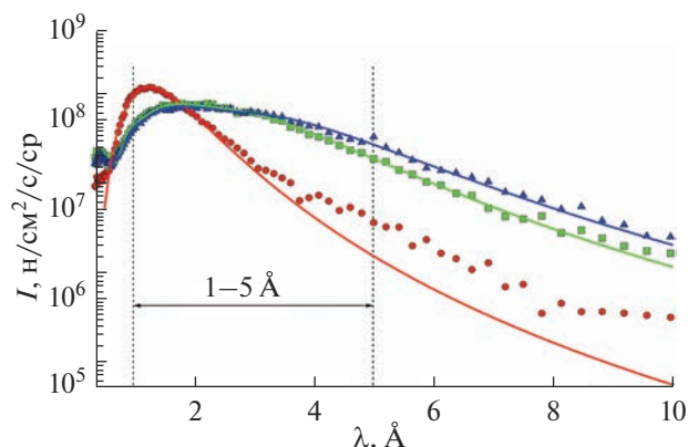
Рис. 3. Спектральная плотность потока нейтронов как функция длины волны для трех типов мишенной сборки компактного источника нейтронов DARIA на расстоянии 10 см от отражателя на входе в нейтронотводы NG: кружки – тепловой замедлитель (PE); квадраты – тепловой (PE) + холодный ( C_9H_{12} ); треугольники – тепловой (PE) + холодный ( p-H_2 ). Сплошные линии – аппроксимация функцией распределения Максвелла. Рабочий спектральный диапазон 1–5 Å выделен вертикальными пунктирными линиями.
