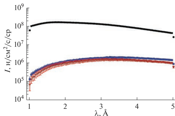
Рис. 5. Изменение спектральной плотности потока для \lambda = 1\text{--}5 Å после нейтронородной системы длиной 21 м: кружки — на выходе из источника; квадраты — на выходе прямого нейтронорода; треугольники — на выходе изогнутого нейтронорода.
