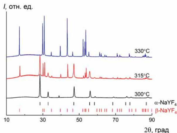
Рис. 1. Дифрактограммы образцов наночастиц \text{NaYF}_4:\text{Yb}(20\%)/\text{Er}(2\%) , полученных при различной температуре синтеза в течение 30 мин.
