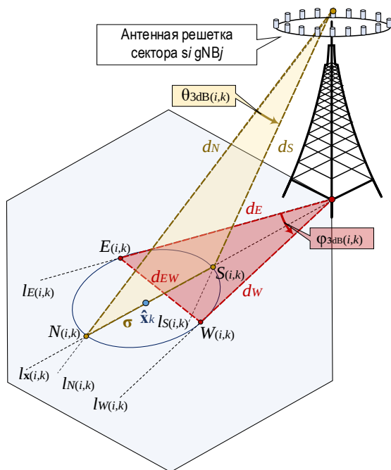
Рис. 5. Настройка ширины луча в горизонтальной и вертикальной плоскостях
