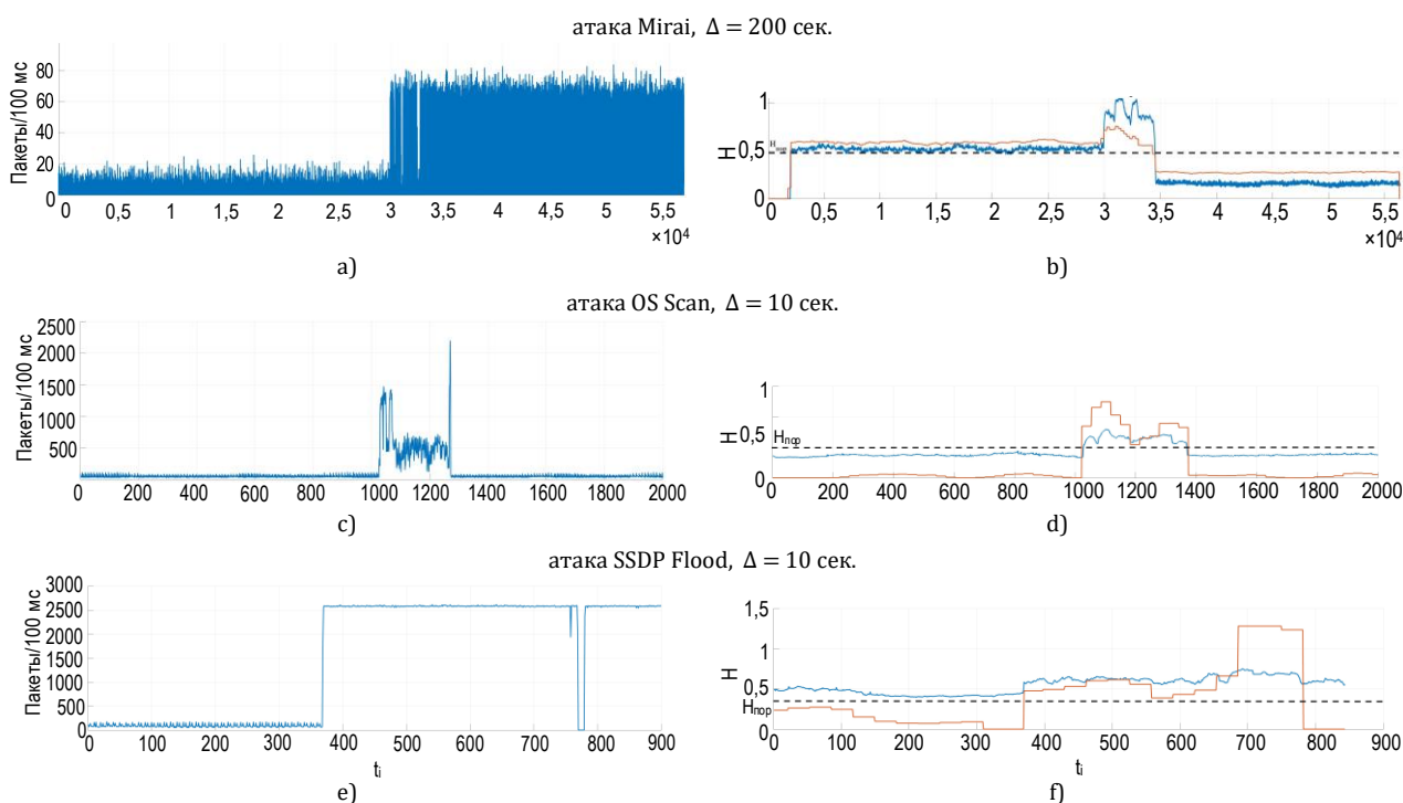
Рис. 5. Оценка H трафика IoT при использовании алгоритмов (1) и (2): а), с), е) фрагмент трафика с атакой; б), d), f) – оценка показателя Херста в скользящем окне
