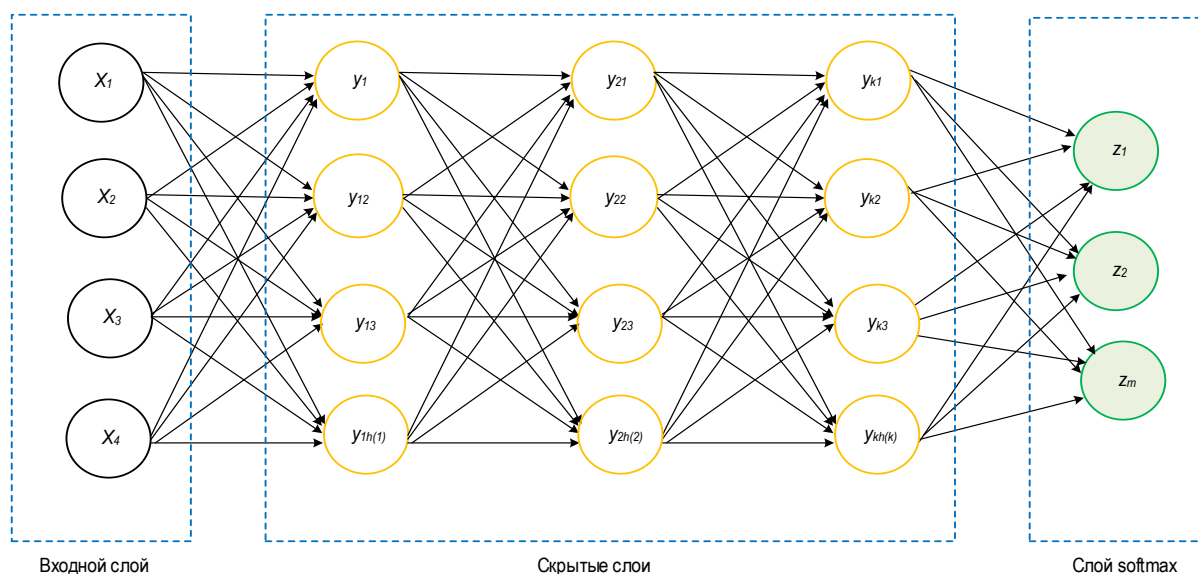
Рис. 3. Модель сети глубокого обучения
