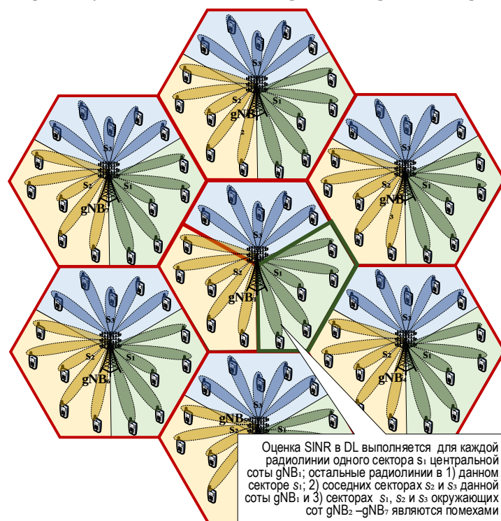
Рис. 1. Сценарий модели диаграммообразования на основе позиционирования
