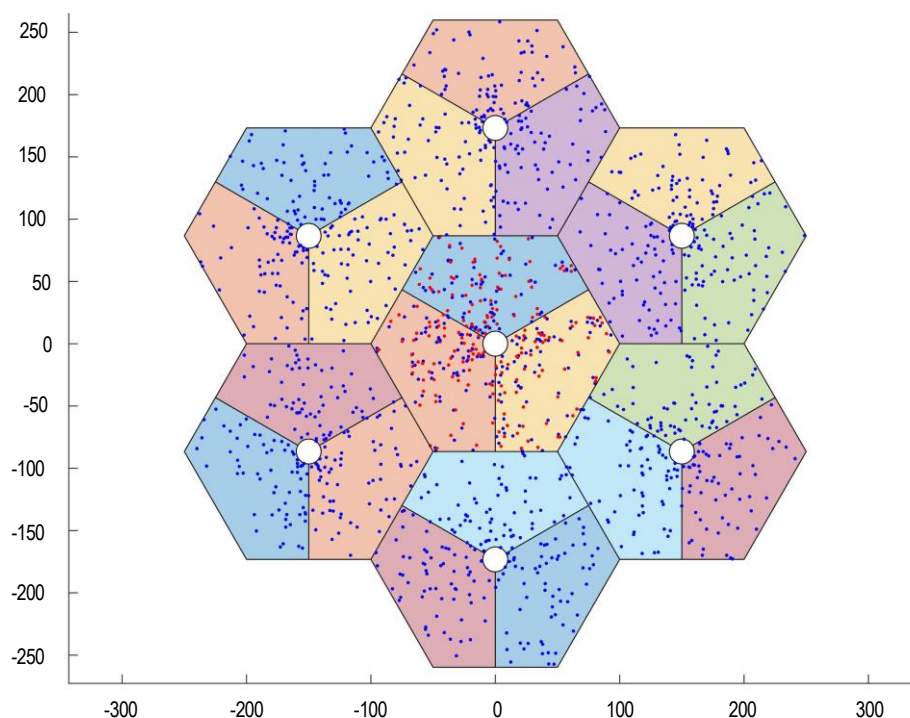
Рис. 8. Сценарий территориального распределения модели совокупности радиолиний
