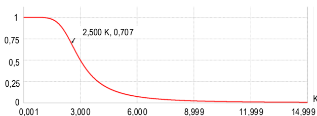
Рис. 13. АЧХ ФНЧ Баттерворта 4-го порядка (2.5 кГц)
