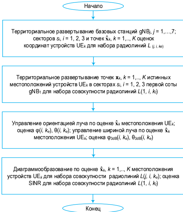
Рис. 7. Процедуры модели диаграммообразования LAB
