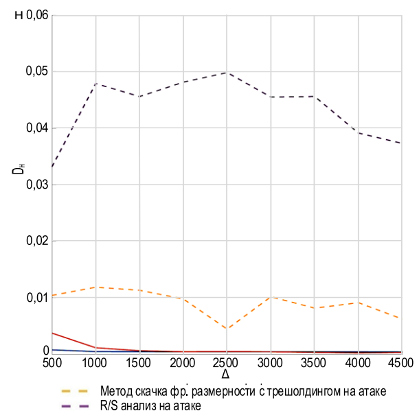
Рис. 3. Зависимости статистических параметров показателя H от размера окна анализа \Delta для дампа нормального трафика IoT и в условиях воздействия атаки Mirai: M_H – слева; D_H – справа
