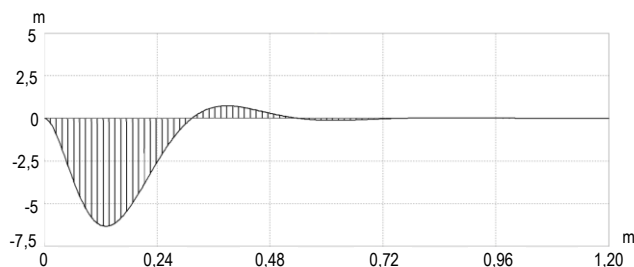
Рис. 15. Отсчеты импульсной характеристики ( f_d = 80 кГц)
