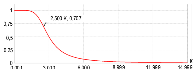
Рис. 17. АЧХ аналогового ФНЧ Баттерворта 4-го порядка с полосой 2.5 кГц и АЧХ КИХ-фильтра
