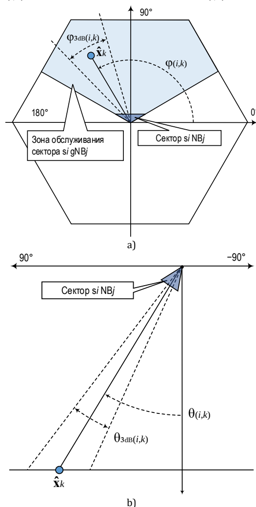
Рис. 4. Характеристика ориентации луча на пользовательское устройство: а) по азимуту (ширина луча в горизонтальной плоскости); б) по углу места (ширина луча в вертикальной плоскости)
