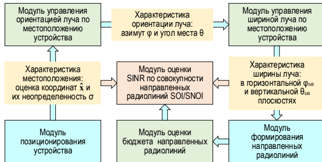
Рис. 2. Функциональная схема модели диаграммообразования LAB
