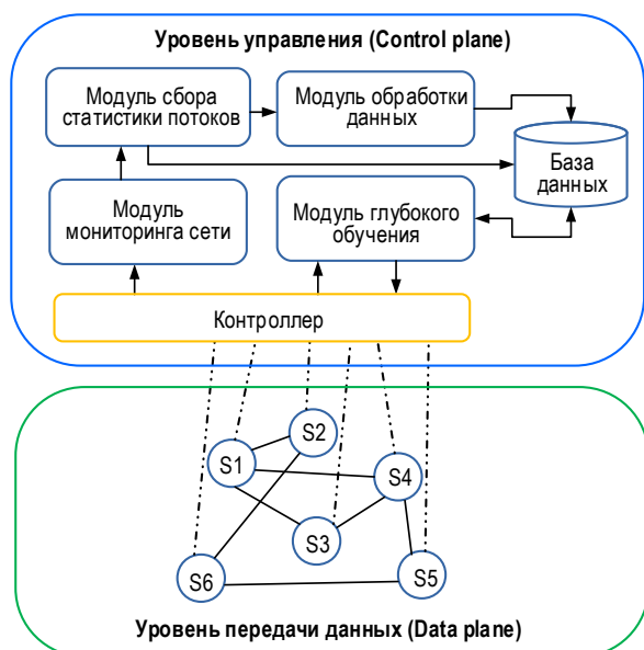
Рис. 1. Архитектура построения модельной сети для классификации приложений трафика
