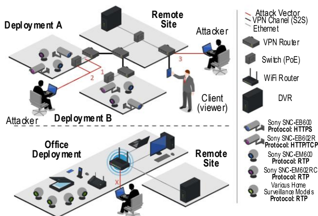
Рис. 1. Топология сети [13]
