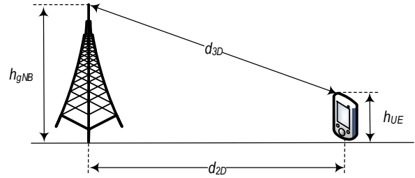
Рис. 6. Сценарий оценки бюджета потерь в направленных радиоперелиниях LOS
