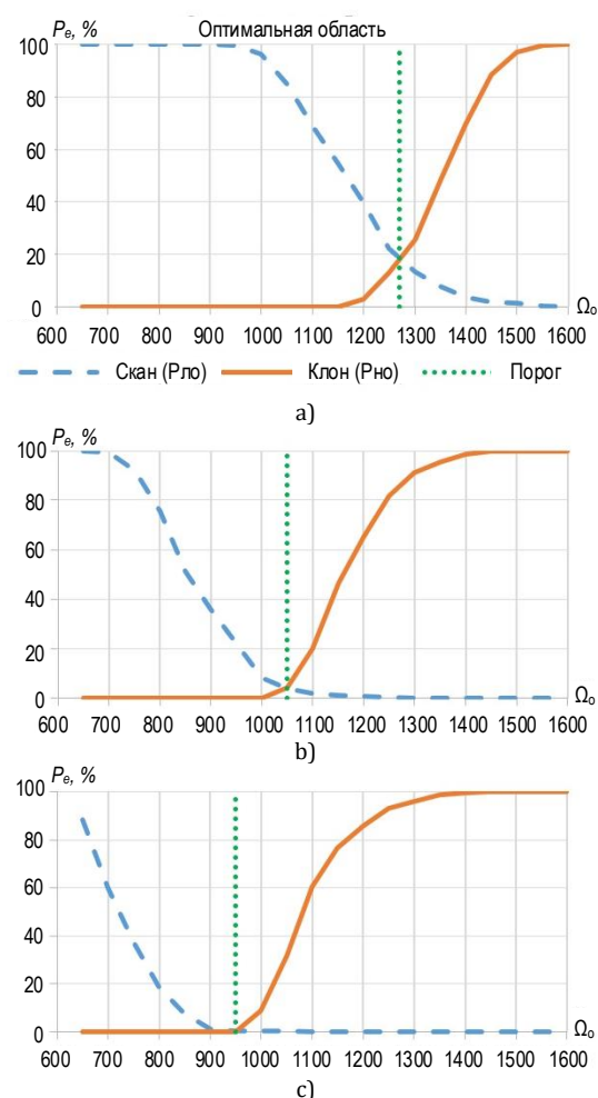
Рис. 6. Зависимость P_m и P_{fa} от величины порога \Omega_0 при разрешении сканирования 200 dpi (a), 300 dpi (b) и 600 dpi (c)
