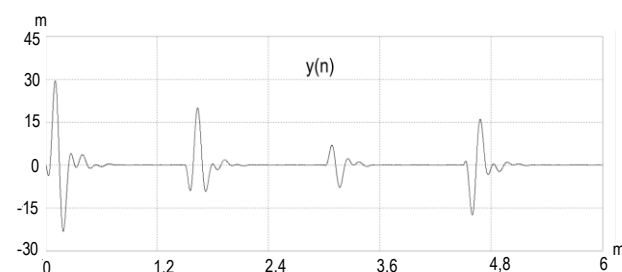
Рис. 26. Суммарный сигнал на выходе модулятора системы передачи данных
