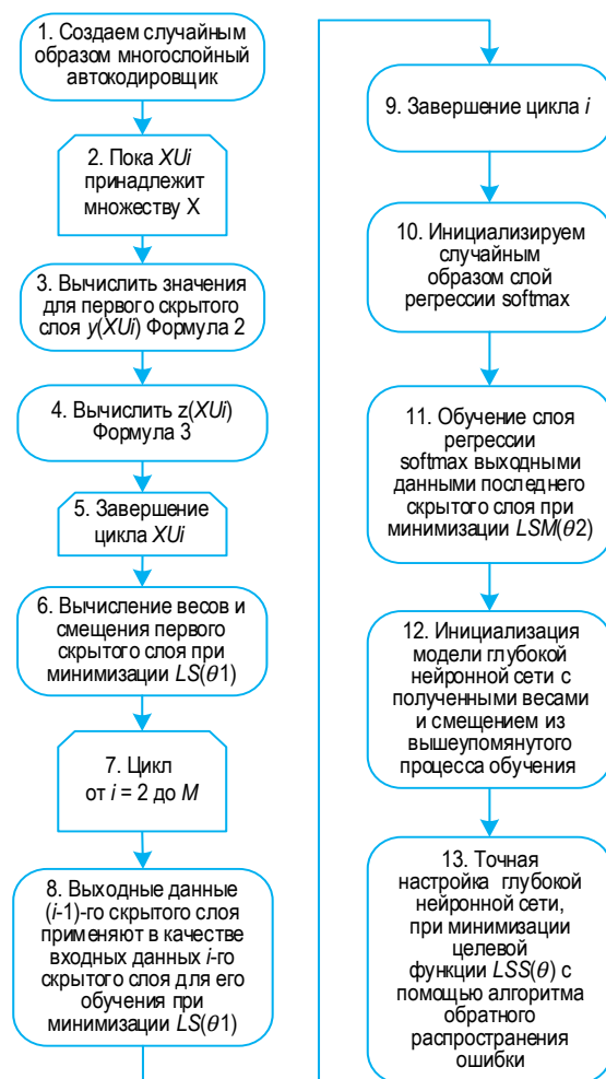
Рис. 4. Алгоритм обучения ГНС
