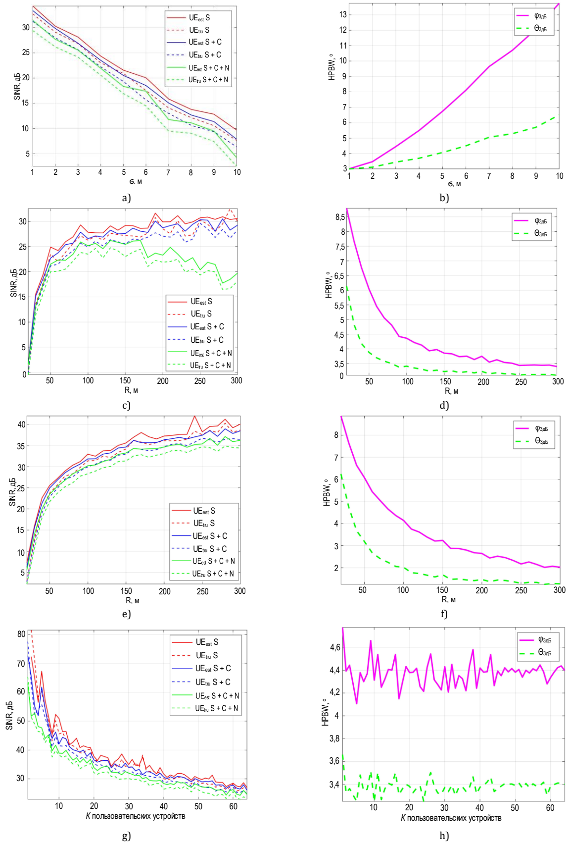
Рис. 9. Зависимость SINR (слева) и HPBW (справа) от точности позиционирования (a, b), размера соты (c, d), размера соты при HPBW_{min} = 1^\circ (e, f) и числа устройств в секторе (g, h)
