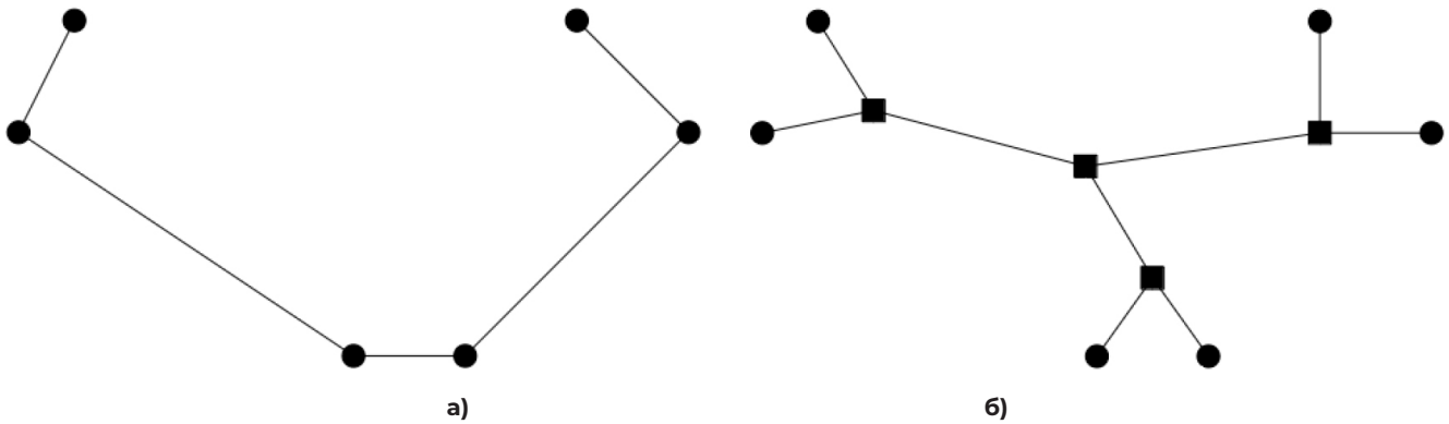
Рисунок 1. Задача Штейнера: а) T \subseteq V ; б) T \neq V
