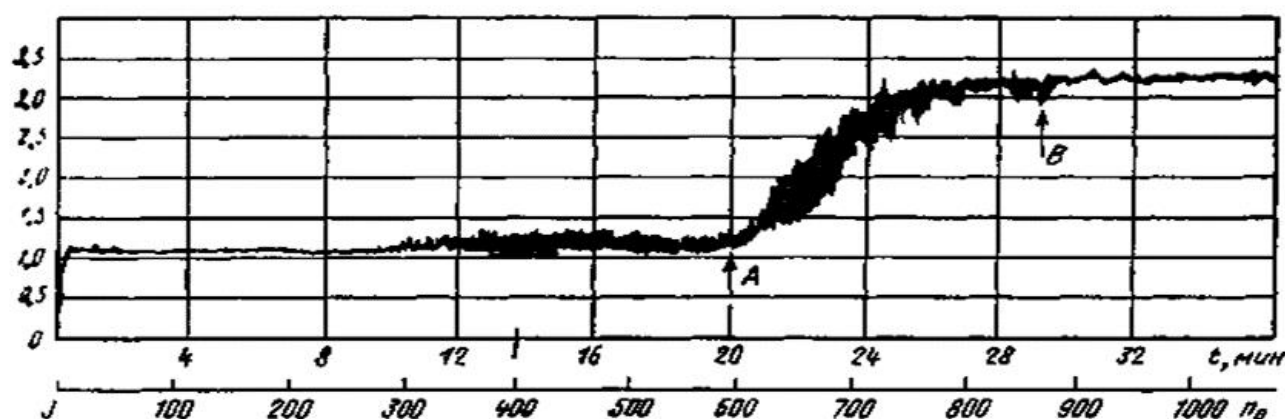
Рисунок 3. Трибограмма испытания образцов при испытаниях на шариковом трибометре.
