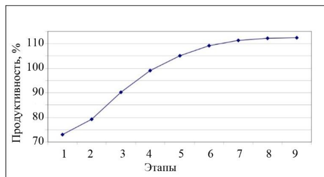
Рис. 2. Изменение коэффициента продуктивности при многократной балансировке выпуска
