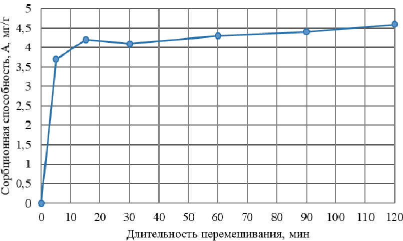
Рис. 3. Кинетическая кривая адсорбции фенола из модельного раствора с концентрацией 100 мг/дм 3 на ТКШ 500 с размером частиц менее 0,315 мм
