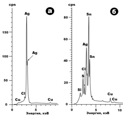
Рис. 19. ЭД-спектры серебряной бусины (а) и использованного при ее изготовлении припоя (б). Fig. 19. ED spectra of a silver bead (а) and the solder used in its manufacture (б).
