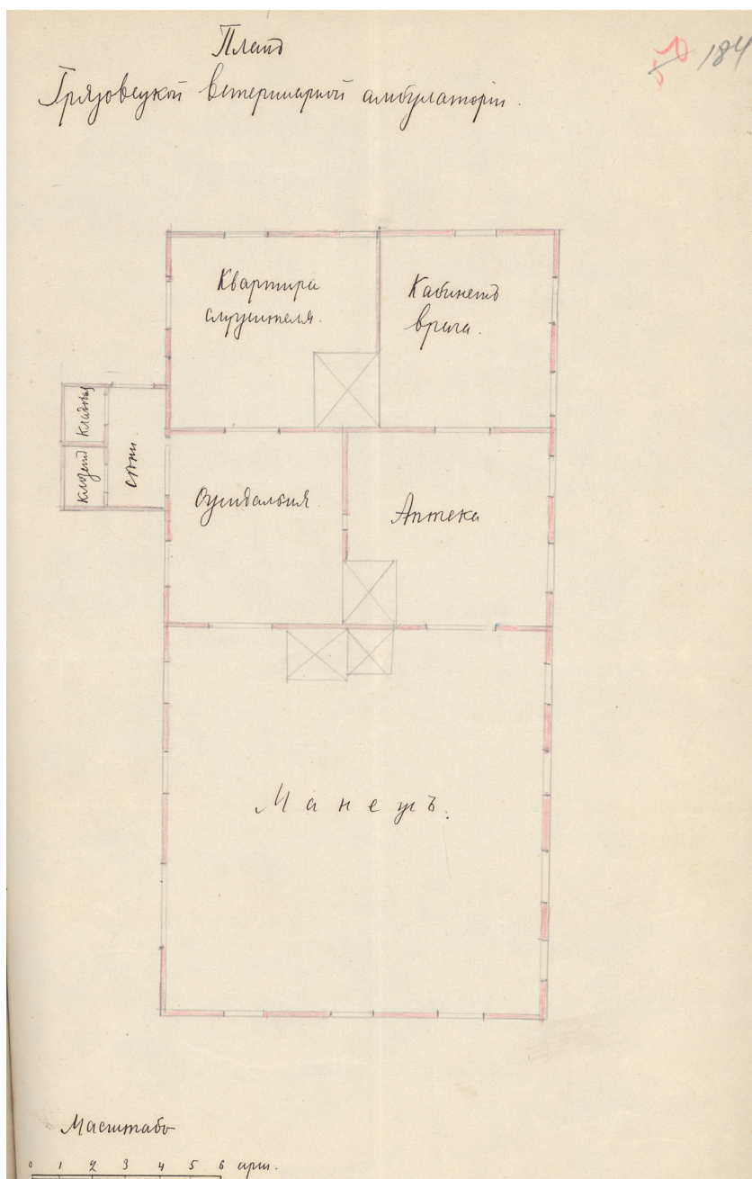
Рис. План ветеринарной амбулатории в г. Грязовце.
