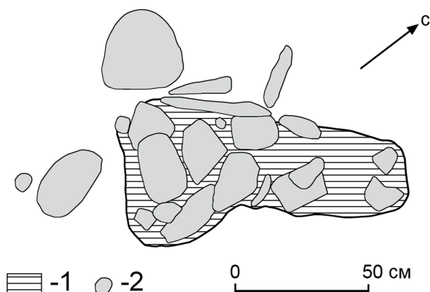
Рис. 5. Горн из каменных плит для производства железа на стоянке Пески IVa. 1 – углистый слой со шлаками; 2 – каменные плиты из уплощенных или расколотых валунов.
