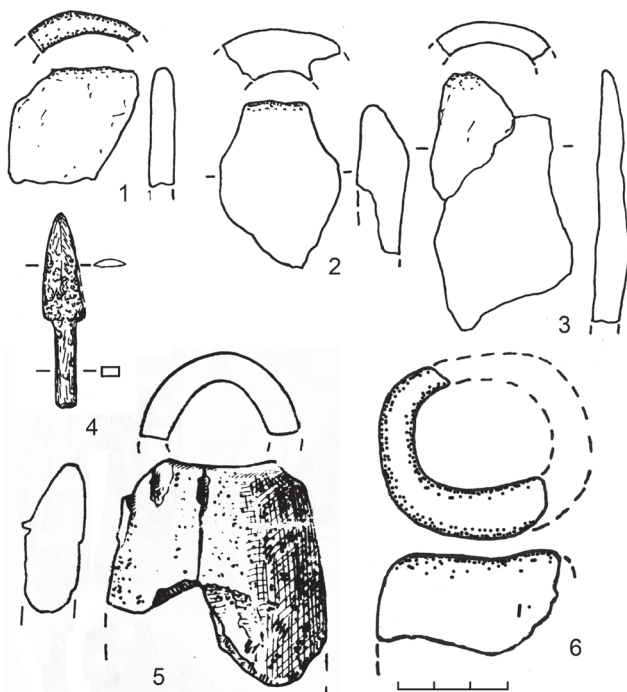
Рис. 4. Керамические сопла (для мехов?) и железный наконечник стрелы со стоянок раннего железного века Карелии: 1–3 – Шуйский Остров I, 4 – Хижозеро I, 5 – Шеттима I [20, рис. 28: 7], 6 – Кудомы XI [20, рис. 28: 8]. Fig. 4. Ceramic nozzles (for bellows?) and an iron arrowhead from the sites of the Early Iron Age of Karelia. 1–3 – Shuisky Island I, 4 – Khizhzero I, 5 – Shettima I [20, Fig. 28: 7], 6 – Kudoma XI [20, Fig. 28: 8].
