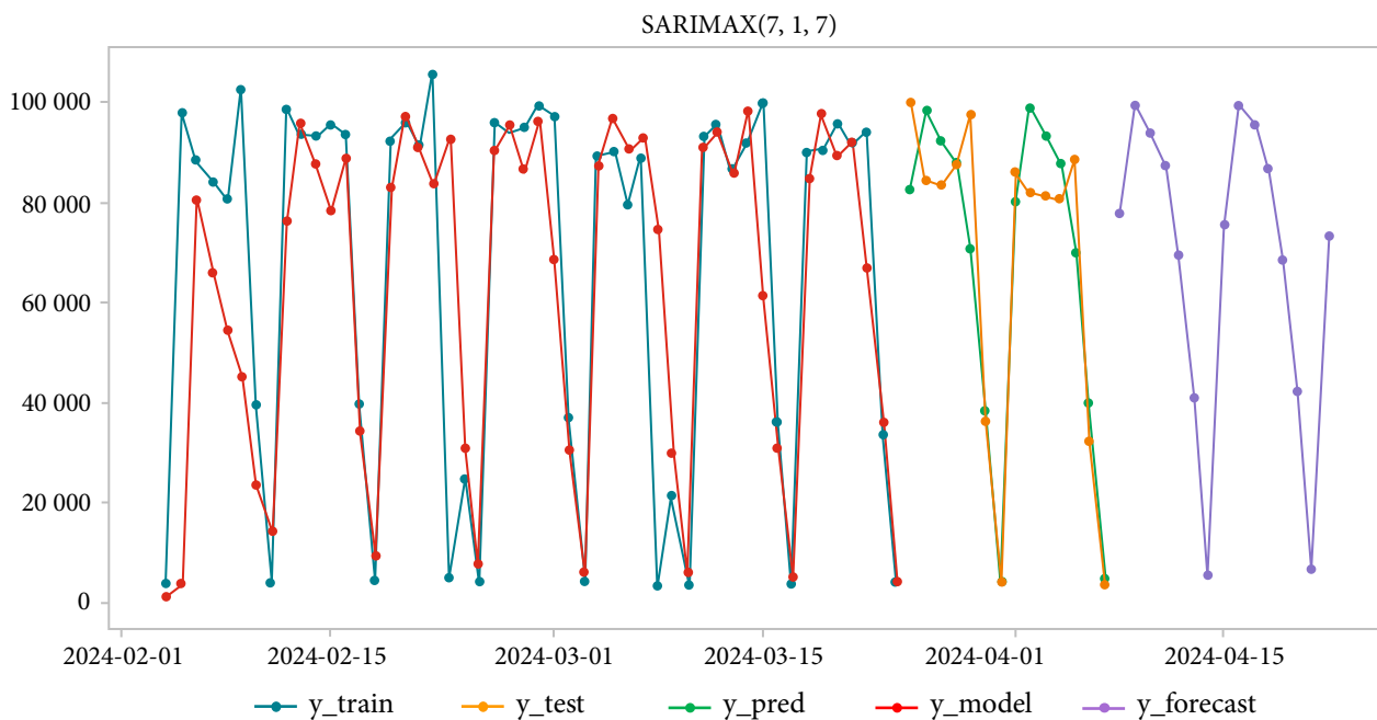
Рис. 11. Модель SARIMAX (7, 1, 7) Fig. 11. SARIMAX Model (7, 1, 7)
