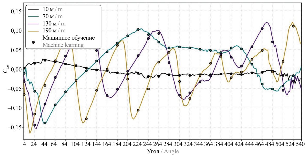
Рис. 14. Сопоставление результатов расчета аэродинамических коэффициентов сил и моментов ( C_x , C_y , C_{Me} ) от параметра угла закручивания формообразующей здания \varphi по результатам CFD-моделирования (сплошные линии) и машинного обучения по модели случайный лес (точки)
