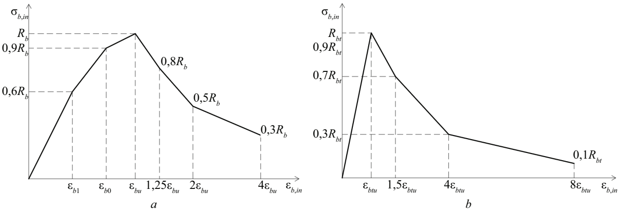
Рис. 2. Диаграмма деформирования бетона: a — при сжатии; b — при растяжении Fig. 2. Compression strain: a — chart for concrete; b — tensile strain
