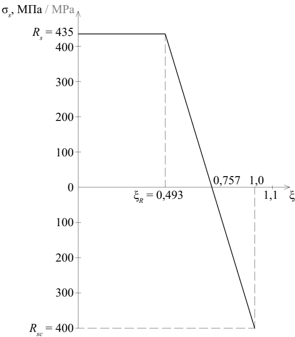
Рис. 1. Линейная аппроксимация нелинейной зависимости \sigma_s от \xi для арматуры класса А500 Fig. 1. Linear approximation of the nonlinear dependence of \sigma_s on \xi for reinforcement class of А500
