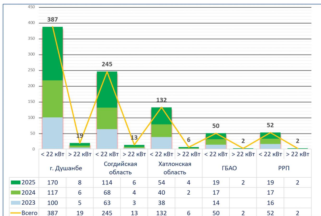
Рисунок 1. Создание специальной зарядной инфраструктуры электроэнергии для электромобилей на первом этапе реализации программы
