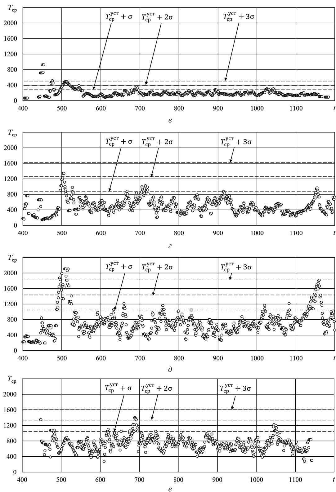
Рисунок 6. Осредненные продолжительности T_{срj} (с) движения автомобилей; а – направление движения 1, б – направление движения 2, в – направление движения 3 (рисунок 2, в), г – направление движения 4, д – направление движения 5, е – направление движения 6 (см. рисунок 2, в); период наблюдения 22 февраля 2023 года Источник: разработано авторами
