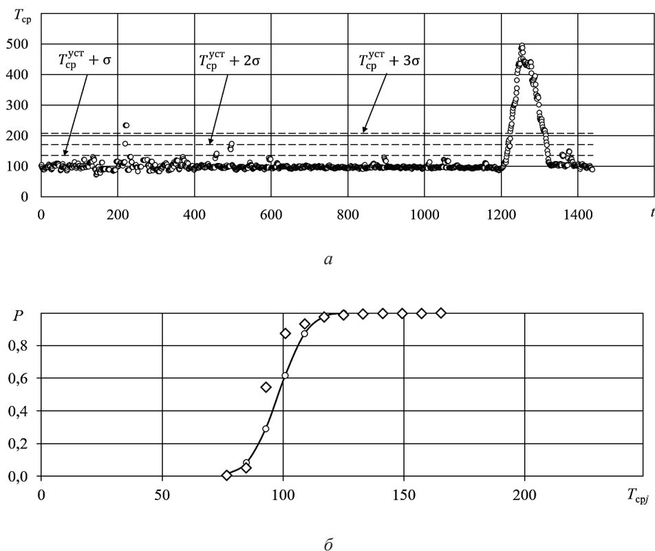
Рисунок 1. Осредненные продолжительности T_{cpj} (с) движения автомобилей (—○—) и пороговые значения (— — —) их отклонения на \sigma , 2\sigma и 3\sigma значений от T_{cp}^{уст} (а); теоретическое (—○—) и эмпирическое (—◇—) распределения P вероятности осредненных продолжительностей T_{cpj} движения автомобилей между рубежами контроля (б); наблюдение в течение суток 9 мая 2022 года
