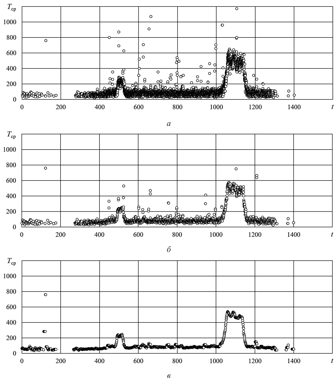
Рисунок 3. Продолжительности T_{срj} (с) движения автомобилей при интервале осреднения \Delta = 10 с и сдвиге \delta = 5 с (а); \Delta = 1 мин и \delta = 30 с (б); \Delta = 10 мин и \delta = 1 мин (в); направление 1 «Восточный обход – улица Старцева», 16 мая 2022 г.
