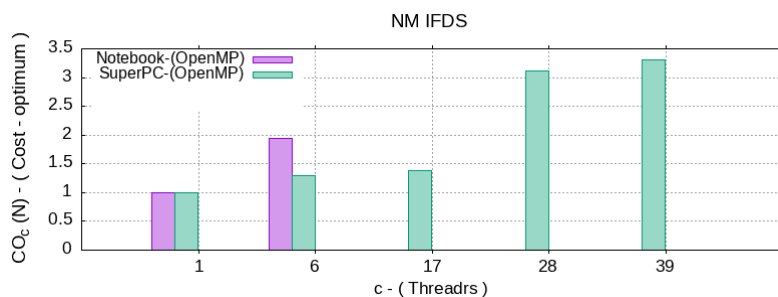
Рис. 5. Стоимостно-оптимальный показатель CO_c(N) при разном c – числе потоков CPU
