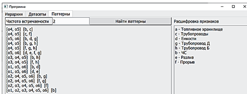
Рисунок 6 – Этап запуска вычислений и получения результирующих паттернов
