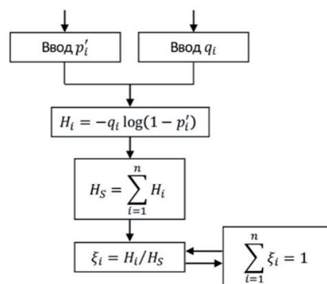
Рисунок 2 – Алгоритм реализации метода
