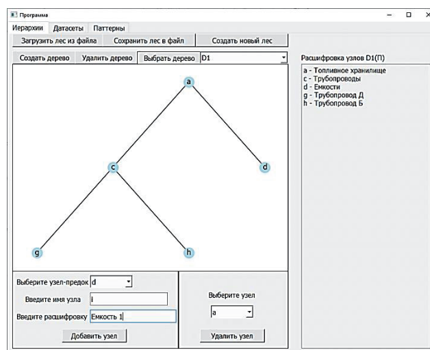
Рисунок 4 – Этап формирования иерархий признаков
