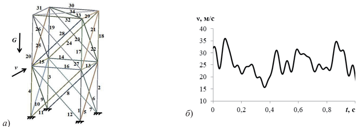
Рисунок 5 – Схема модельной задачи: а) конфигурация стержневой системы; б) характерный фрагмент изменения скорости ветра v
