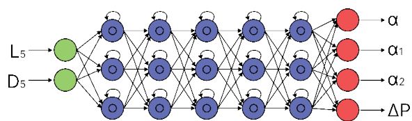
Рисунок 8 – Схема модели, предикторами которой являются линейные параметры диффузора
