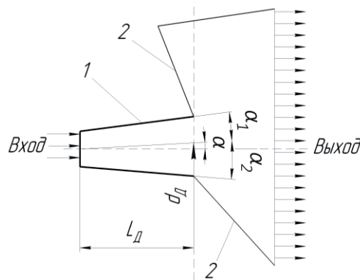
1 – диффузор, 2 – элементы корпуса
