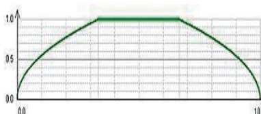
Рисунок 8 – Функция принадлежности классу с фронтами обратной параболы
