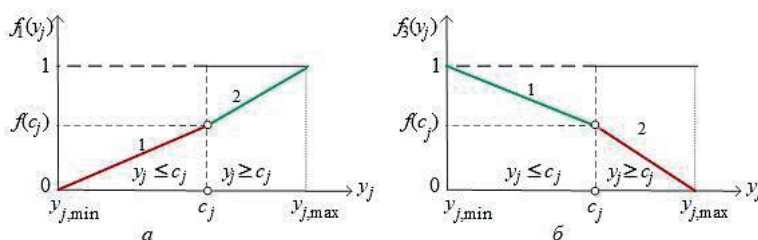
Рисунок 3 – а) оценочная функция f_1 , б) оценочная функция f_3
