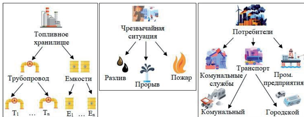
Рисунок 1 – Иерархии признаков
