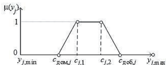
Рисунок 2 – Модель расплывчатой нормы
