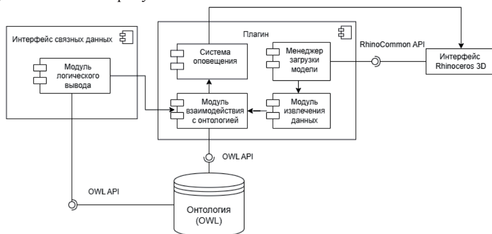
Рисунок 4 – Диаграмма компонентов системы анализа градостроительных проектов
