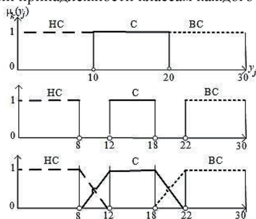
Рисунок 11 – Варианты границ между классами
