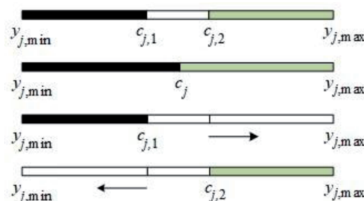
Рисунок 1 – Четыре варианта задания нормы
