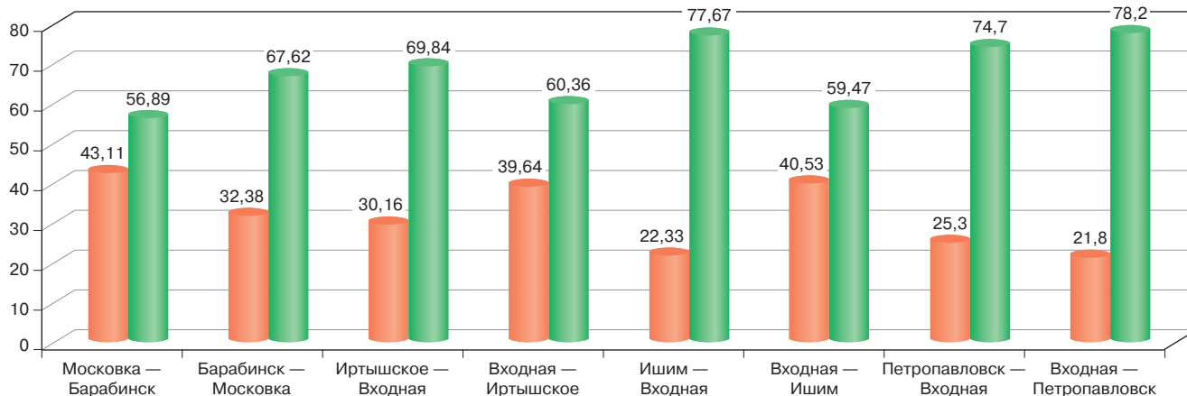
Рис. 3. Доля использования режимов системы автоведения электровозов серии 2ЭС6:
