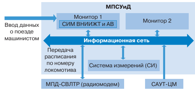
Рис. 1. Структура информационного взаимодействия СИМ-ВНИИЖТ и АВ с аппаратурой электровоза
