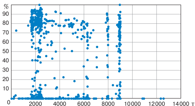
Рис. 4. Результаты усреднения данных об использовании режима автоведения на тяговых плечах Омск — Иртышское — Омск
