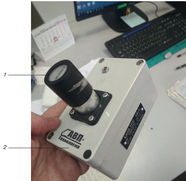
Рис. 16. Картридж с информацией и считывающее устройство ИСАВП-РТ компании АВП «Технология»: 1 — съемный носитель (картридж); 2 — считывающее устройство
