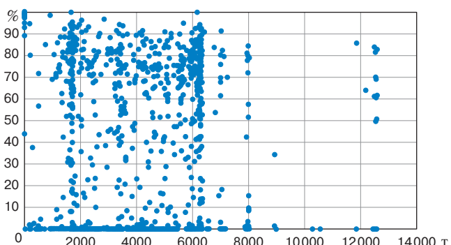
Рис. 5. Результаты усреднения данных об использовании режима автоведения на тяговых плечах Омск — Барабинск — Омск
