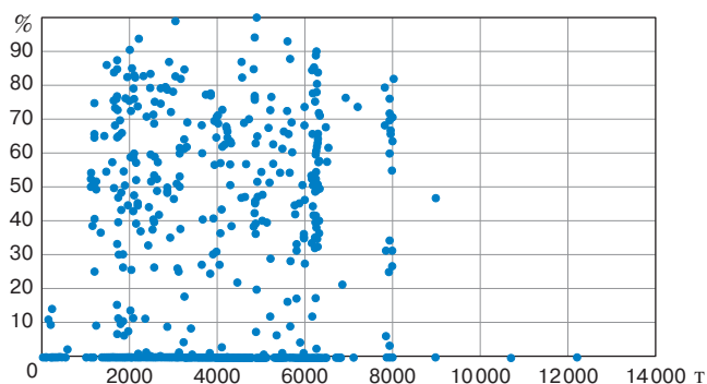
Рис. 6. Результаты усреднения данных об использовании режима автоведения на тяговых плечах Омск — Ишим — Омск
