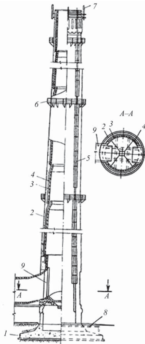
Рис. 1. Схема железобетонной дымовой трубы: 1 — фундамент; 2 — ствол; 3 — футеровка; 4 — теплоизоляция; 5 — ходовая лестница; 6 — световоронная площадка; 7 — молниеотвод; 8 — заземление молниеотвода; 9 — вход газохода
