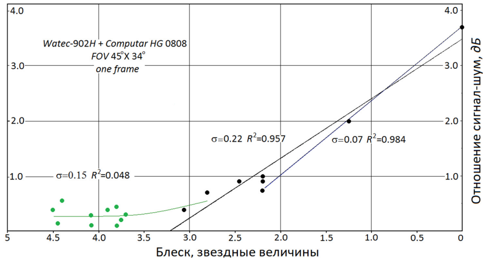
Рис. 2. Соотношение между блеском звезд и их яркостью на изображении
