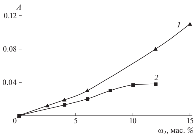
Рис. 3. Концентрационная зависимость оптической плотности для систем ГПЦ–вода/этанол с содержанием этанола 9 (1) и 80 об. % (2). \lambda = 550 нм.
