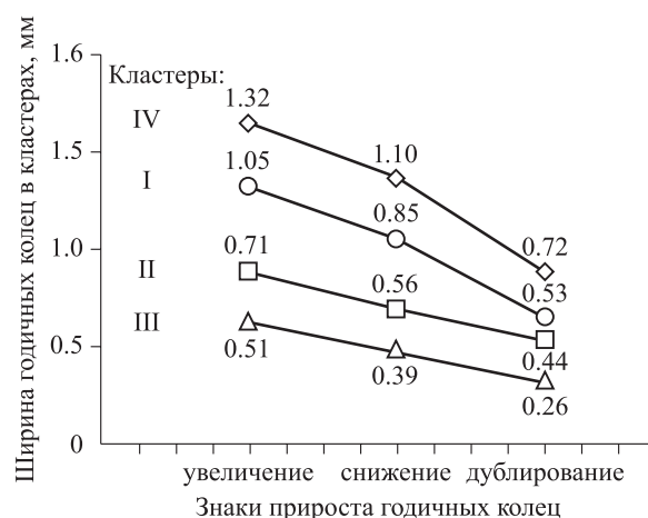
Рис. 3. Ширина годичных колец по знакам радиального прироста в кластерах болотных сосняков.
