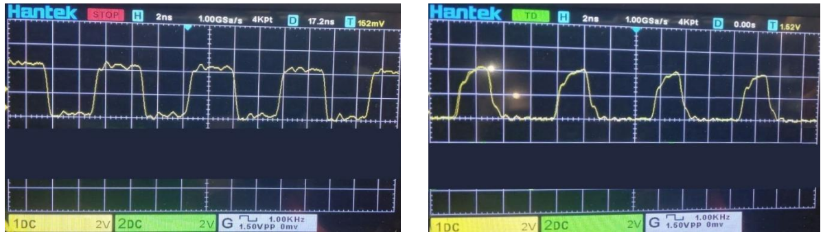
Рисунок 9 – Выходной сигнал: D=50% (а), D=38% (б)
