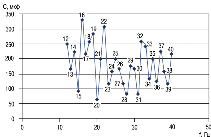
Рис. 1. Результаты исследования изменения емкостной составляющей полного сопротивления экстракционного раствора в зависимости от частоты электромагнитного поля с фиксированной напряженностью H = 0,5 \text{ А/м}
