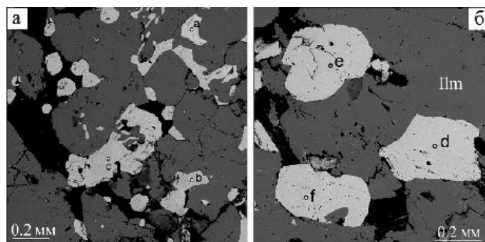
Рис. 5. Зерна красновато-коричневого фторкальциопироклора (a, d, e, f) и ферсмита (c, b) в агрегате ильменита (Ilm) с полевым шпатом (черное).
