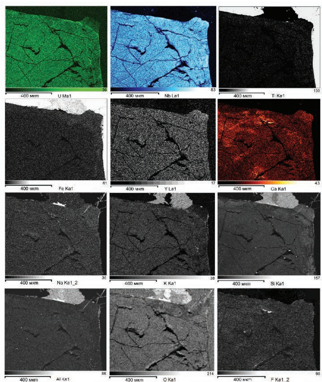
Рис. 4. Карты распределения элементов в исследованном участке «уранпироксена».
