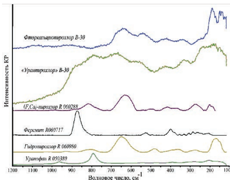
Рис. 6. КР-спектры фторкальциопироклора и «уранпироклора» в сопоставлении с КР-спектрами (F-Ca)-пироклора, ферсмита, гидропироклора и уранофана из базы RRUFF ( http://rruff.info ).
