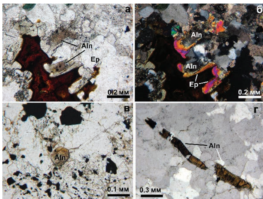
Рис. 9. Кластогенный алланит (Aln): а, б – с каемками эпидота (Ep) в ассоциации с гидроксидами железа в песчаном известняке (а – без анализатора, б – с анализатором); в – кристалл алланита в олигомиктовом песчанике; г – брекчированный алланит в кварц-полевошпатовой жилке. Проходящий свет. Удоканское месторождение.
