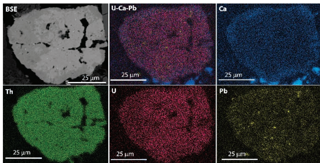
Рис. 7. BSE изображение неоднородного зерна «торита» с включениями сульфида свинца и каймой, обогащенной Ca, и распределение основных элементов. Ункурское месторождение.
