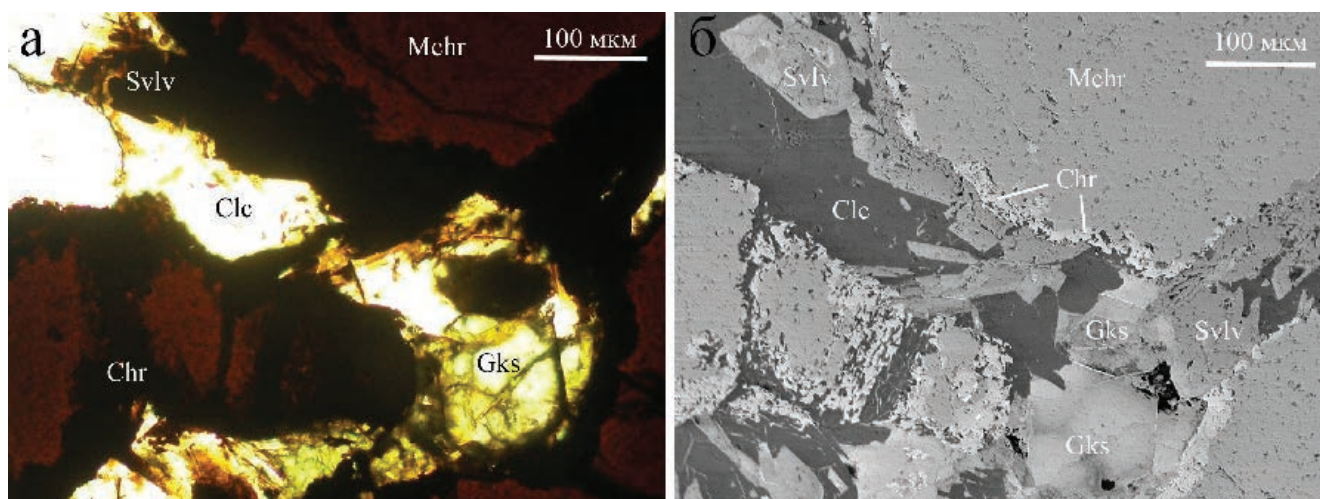
Рис. 5. Прожилок, выполненный поздними минералами, в хромитите Бурхойлинского участка: а – оптический микроскоп, без анализатора; б – СЭМ-фото в режиме отраженных электронов.
