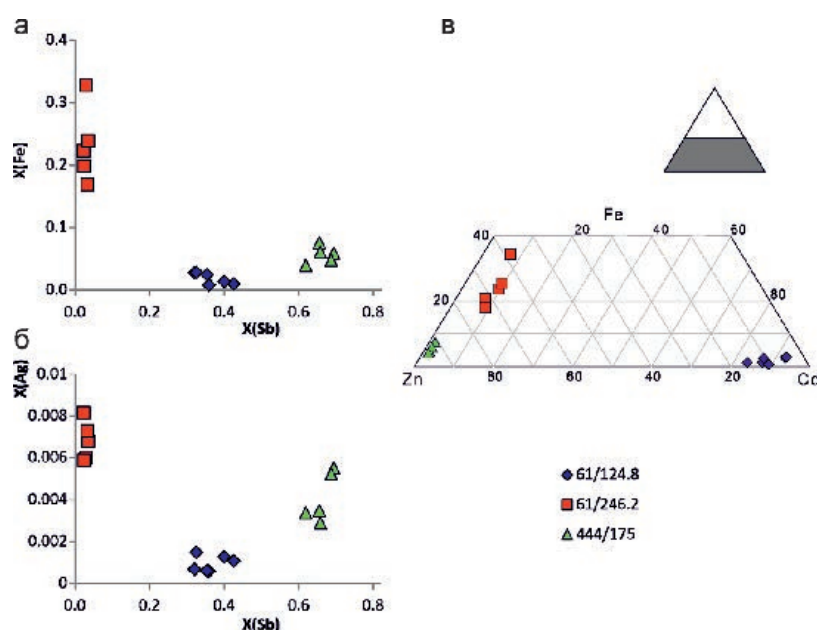
Рис. 6. Диаграммы X(Sb)–X(Fe) (а), X(Sb)–X(Ag) (б) и Fe–Zn–Cd (в) для блёклых руд Томинского месторождения. Fig. 6. X(Sb) vs. X(Fe) (a), X(Sb) vs. X(Ag) (b) and Fe–Zn–Cd ternary (c) diagrams for fahlores of the Tomino deposit.
