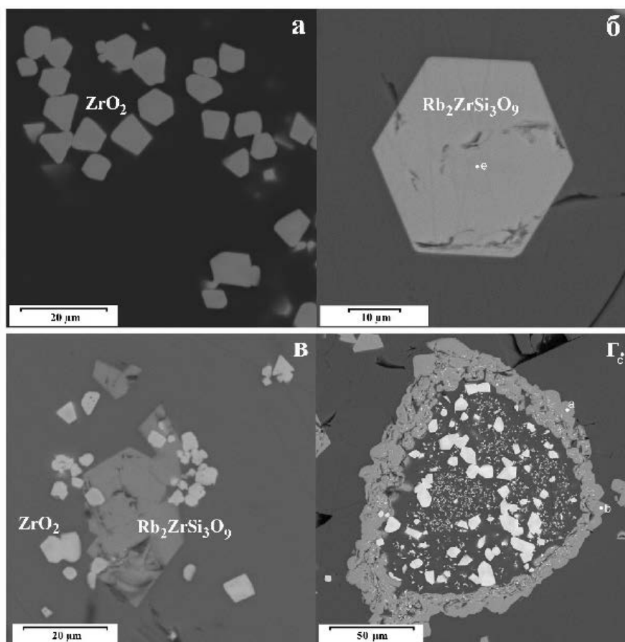
Рис. 1. Электронные изображения кристаллов бадделеита (а, в, г) и цирконосилката Rb (б–г) в синтезированных образцах. Точки а, б, с, е – анализируемые участки.
