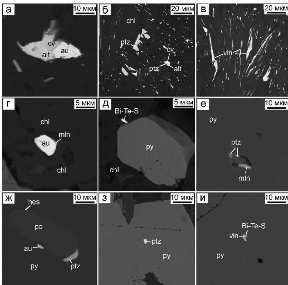
Рис. 9. Морфология самородного золота и теллуридов в слюисто-хлоритовой (а–д) и пирит-пирротитовой (е–и) ассоциациях: а – сросток самородного золота (au), алтаита (alt) и калаверита (cv) среди нерудных минералов; б – сросток калаверита, петцита (ptz) и алтаита и включения петцита в хлорите и слюде (chl); в – включения вольтинскита (vln) по спайности в хлорите и слюде; г – включения самородного золота с каймой мелонита (mln) в хлорите; д – удлиненное зерно минерала Bi-Te-S на контакте пирита (py) и нерудной массы; е – вытянутые включения петцита и мелонита в пирите; ж – включения самородного золота, петцита и гессита (hes) по контурам овального включения пирротина (po) в пирите; з – угловатое включение петцита в пирите; и – сросток вольтинскита и минерала Bi-Te-S в пирите. BSE фото.
