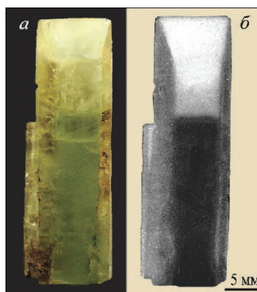
Рис. 13. Вид сечения зонально-секториального берилла № Св-82 (а) и его радиография (б), по (Попова, 1995).
