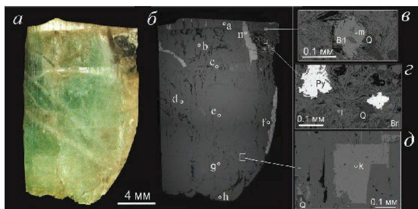
Рис. 3. Вид сечения (а) и фото в отраженных электронах (б) берилла № 46 с минеральными включениями (в–д). Fig. 3. Section view (a) and BSE photo (б) of beryl no. 46 with mineral inclusions (в–д).
