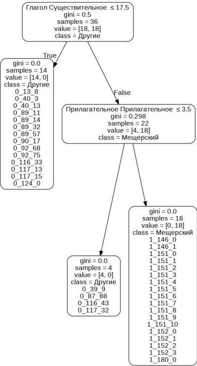
Алгоритм 2 Algorithm 2
