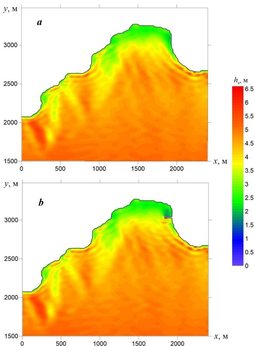
Рис. 3. Значимые высоты волн в бухте Ласпи при штормах, возможных 1 раз в 25 лет, без учета гидротехнического сооружения (a), с учетом гидротехнического сооружения (b)
