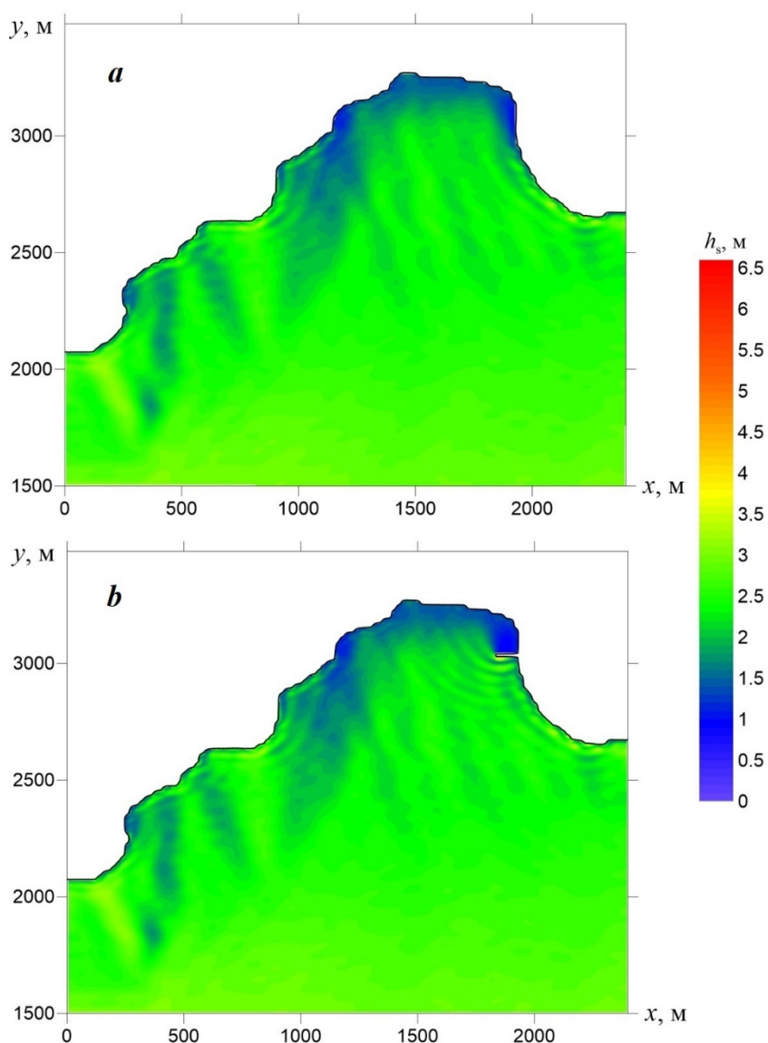
Рис. 2. Значимые высоты волн в бухте Ласпи при штормах, возможных 1 раз в год, без учета гидротехнического сооружения ( a ), с учетом гидротехнического сооружения ( b )
