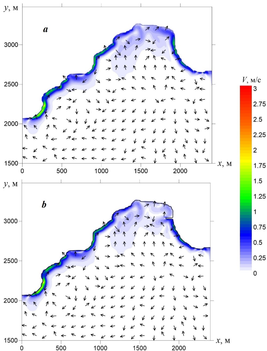
Р и с . 4 . Волновые течения в бухте Ласпи при штормах, возможных 1 раз в год, без учета гидротехнического сооружения (а), с учетом гидротехнического сооружения (b)
