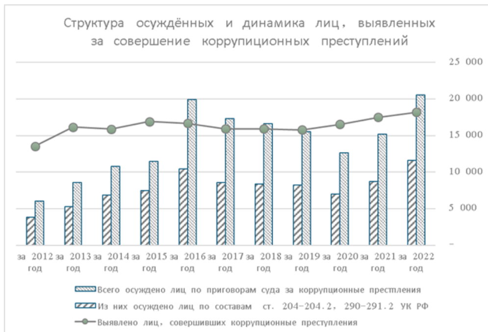
рис.1. Трёхгодичные циклы.
