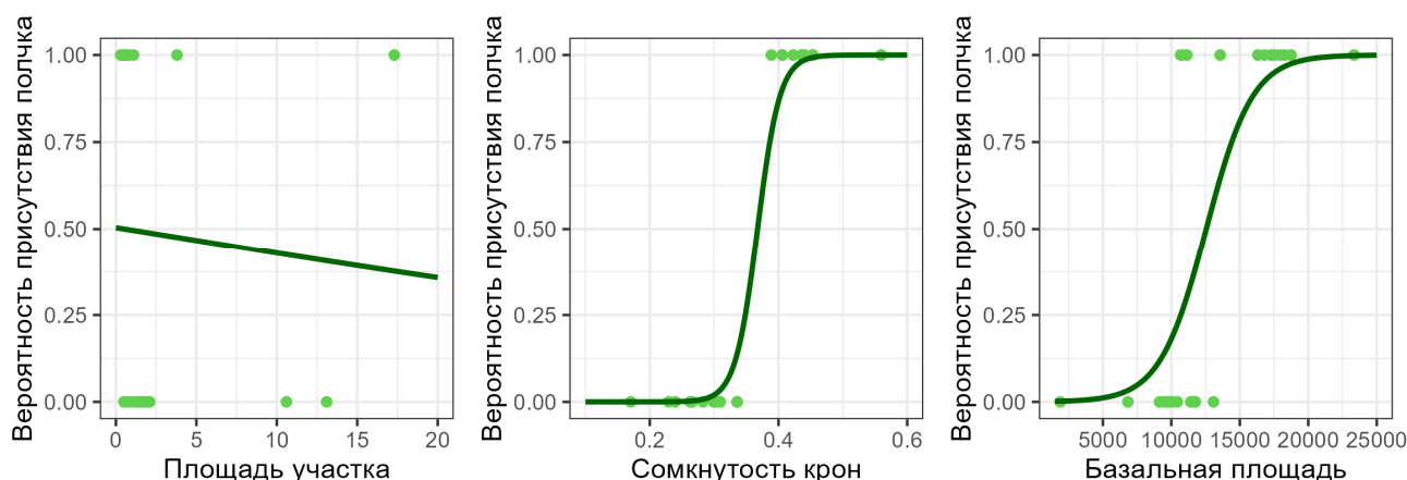
Рис. 2. Вероятность присутствия сони-полчка в зависимости от площади участка, сомкнутости крон и базальной площади деревьев. Точками отмечено присутствие/отсутствие сони, кривая отражает соответствующую модель логистической регрессии
