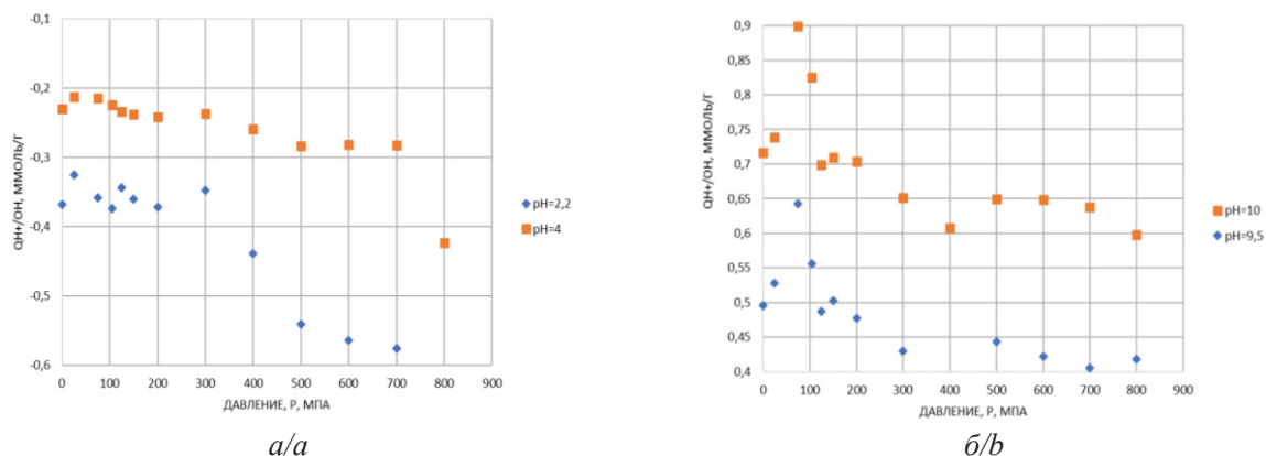
Рис. 5. Зависимость анионообменной емкости Q_{OH^-/H^+} бентонитовой глины от давления при pH=2,2 и pH=4 (а) и зависимость катионообменной емкости Q_{H^+/OH^-} бентонитовой глины от давления при pH=10 и pH=9,5 (б) Fig. 5. Dependence of the anion exchange capacity Q_{OH^-/H^+} of bentonite clay on pressure at pH=2,2 and pH=4 (a) and dependence of the cation exchange capacity Q_{H^+/OH^-} of bentonite clay on pressure at pH=10 and pH=9,5 (b)
